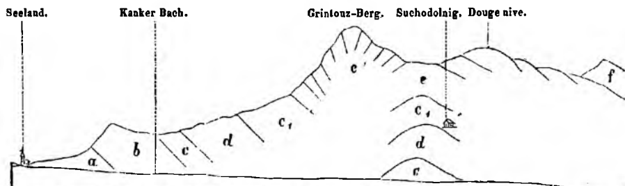
N. a Gailthaler Schiefer und Sandstein. b Gailthaler Kalkstein. c Werfener Schiefer und Sandstein. c 1 Guttensteiner, veränderter Kalkstein. d Porphyr. e Hallstätter Schichten. f Dachsteinkalk.
