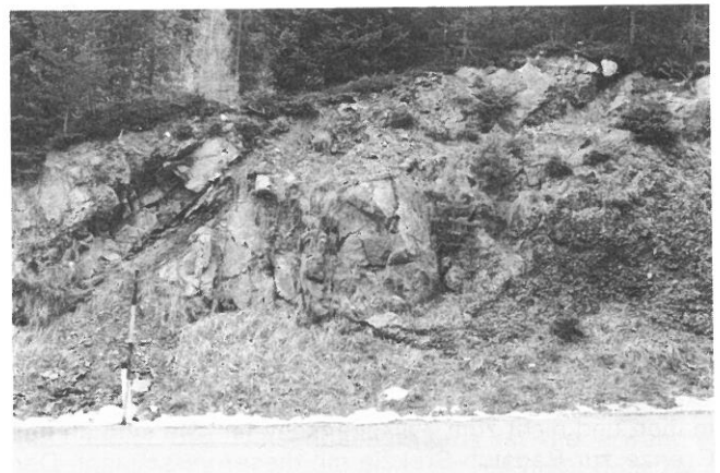
Abb. 4: Profilausschnitt des Straßenaufschlusses durch den oberen Teil der Nötsch Formation an der Straße von Pölland auf die Windische Höhe. Wechsellagerung von Siltsteinen, Sandsteinen und Konglomeraten.
