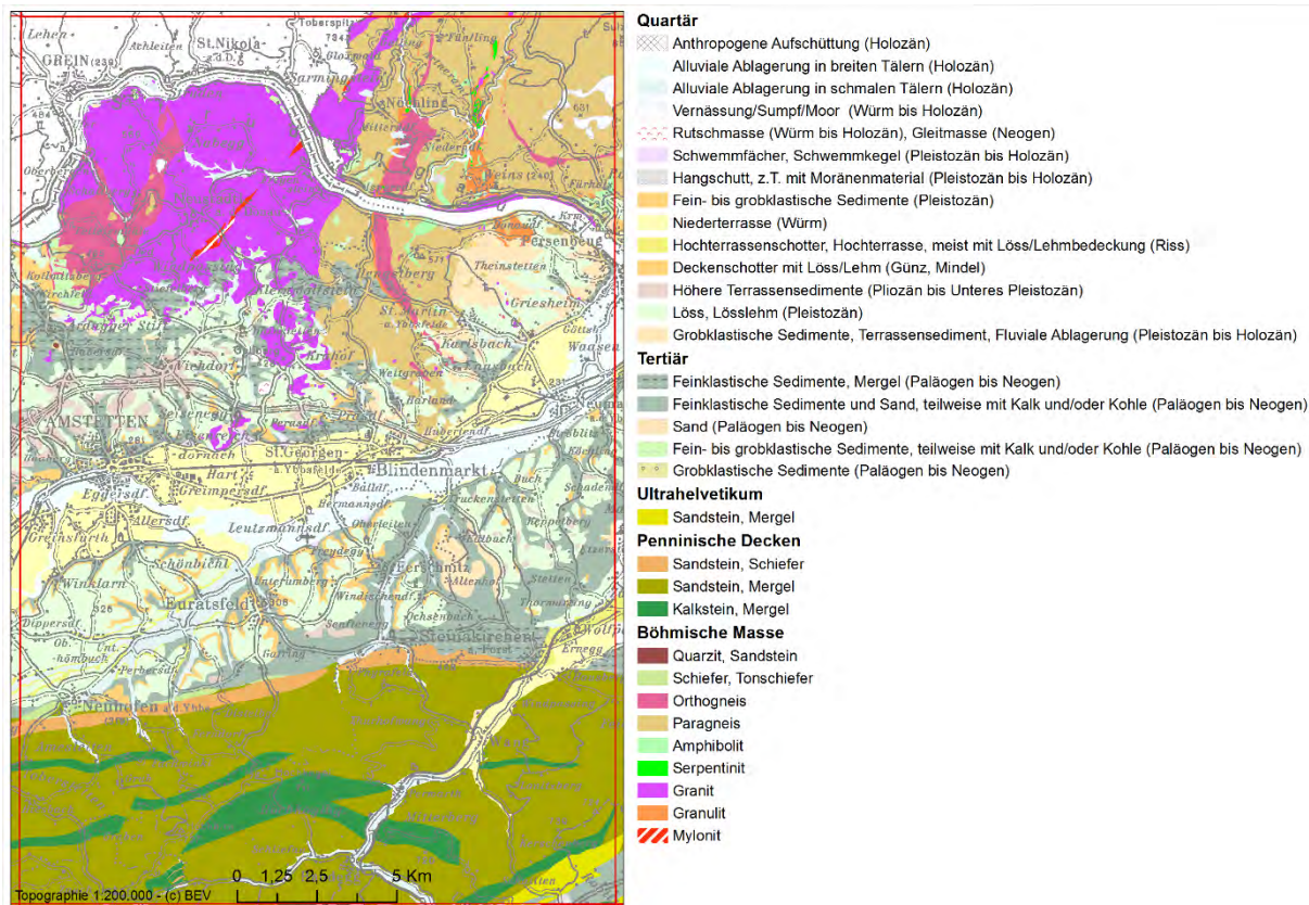
Abb. 5: Beispielhafter, verkleinerter Ausschnitt aus der GIS-basierten, digitalen, angewandt-geologischen Arbeitskarte „AngedAN“ im Maßstab 1:50.000.
