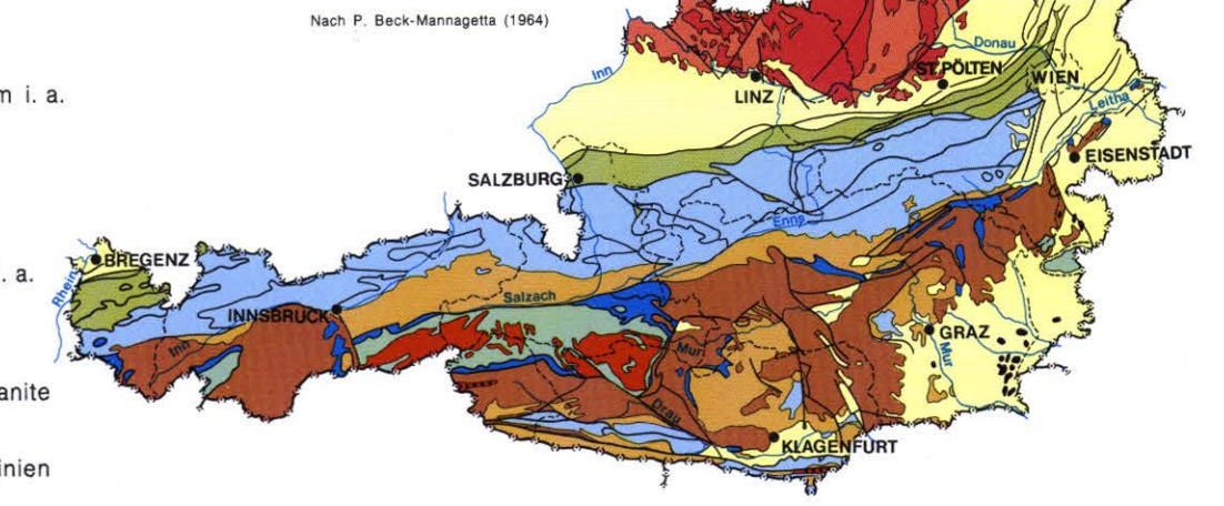
Geologische Übersichtskarte
