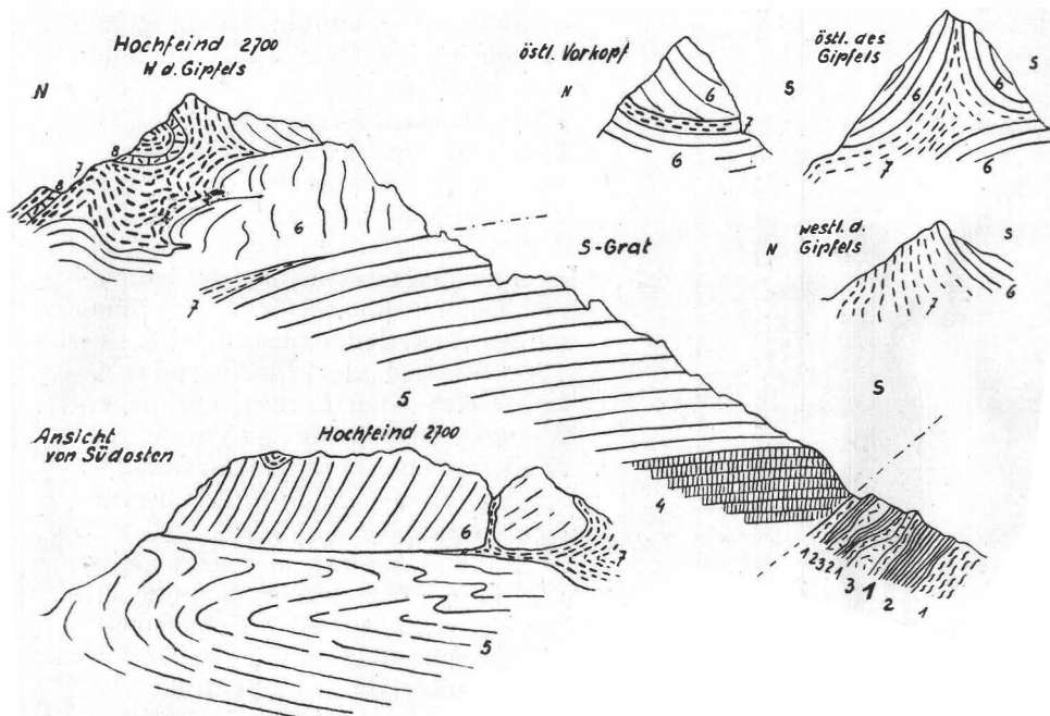
Fig. 21. 1. Grünlicher und grauer Phyllit; 2. Kalkglimmerschiefer; 3. gelbgrauer, zerhackter Dolomit; 4. dolomitische Raibler; 5. Hauptdolomit, gleichmäßig gebankt; 6. Hauptdolomit, undeutlich gebankt; 7. dunkle Schiefer und Kalkschiefer des Lias; 8. Bank von dunklem Dolomit.
