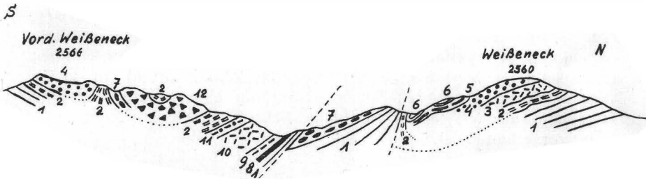
Fig. 16. Der Lias am Gipfel des Weißenecks. 1. Hauptdolomit; 2. kalkig-sandige Tonschiefer, zum Teil mit etwas schwarzem Marmor und phyllitischen Dolomitreccien; 3. grauer Dolomit; 4. gelbliche reine Dolomitreccie; 5. Breccie mit Quarzitschollen von über 1 m; 6. Kalkglimmerschiefer; 7. Dolomitreccie mit viel Phyllitschollen; 8. schwarzer, verwitterter brauner Dolomit; 9. schwarzer, sandiger Tonschiefer; 10. graue reine Dolomitreccie; 11. grünlicher serizitischer Schiefer mit einzelnen Dolomitbrocken; 12. grobe gelbliche Dolomitreccie, Quarzit selten.
