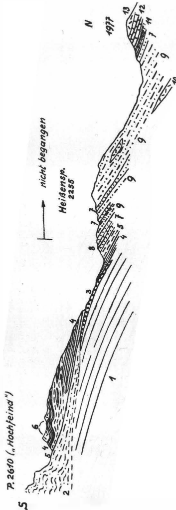
Fig. 12. Schnitt von P. 2610 (Hochfeind) nach Nord. 1. Hauptdolomit; 2. Liaschiefer mit viel Breccien; 3. gelbe, reine Dolomitreccie; 4. Kalkgimmerschiefer; 5. grauer Phyllit; 6. gelblicher, stark zerbrochener Dolomit; 7. heller Serizitquarzit; 8. lichtgrauer Marmor; 9. Kristallin; 10. Dolomit ähnlich 6.; 11. Rauhacke; 12. grauer Bändermarmor; 13. heller Dolomit.
