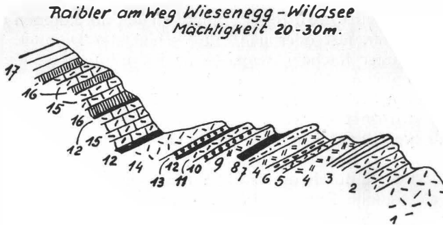
Fig. 6. Raibler Schichten am Weg Wiesenegg-Wildsee. 1. mächtiger heller ungeschichteter Dolomit (Wetterstein); 2. desgleichen gelblich verwittert und gebankt; 3. gelb bis gelbbraun verwitterter Dolomit; 4. grauer, schmutzig verwitterter Dolomit; 5. desgleichen hellgrau verwittert; 6. lichtgrüner Schiefer; 7. graue kieselige Schieferbank; 8. schwarzer, zum Teil bänderiger Tonschiefer; 9. schwarzer, braun und gelb verwitterter Dolomit; 10. gelblichgraue, reine Dolomitbreccie; 11. hellgrauer Dolomit; 12. schwarzer Tonschiefer; 13. gelbe Dolomitbreccie mit einzelnen lichten Schieferschollen; 14. hellgrauer Dolomit, zum Teil brecciös, zum Teil gebändert; 15. dunkle gebankte, zum Teil brecciöse, zum Teil gebänderte Dolomite, schmutzig verwittert; 16. dunkle, weiß anwitternde Dolomitbänke; 17. Übergang in Hauptdolomit, darin auch bläulich verwitterte Dolomitbänke.
