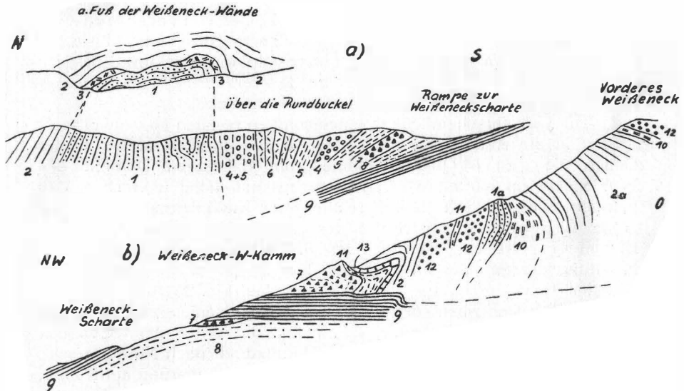
Fig. 25. a) Schnitt durch das Kar westlich des Weißenecks und b) Weißeneck-Westkamm. 1. Heller Quarzit und Quarzitschiefer; 2. bankiger Dolomit; 2a. Hauptdolomit; 3. gelbliche Dolomite und Breccien; 4. gelbliche Dolomittbreccien; 5. graubraune, etwas sandige Schiefer; 6. schwarzer, blaugrau anwitternder Dolomit; 7. Dolomittbreccien mit Schieferschollen; 8. grauer Phyllit; 9. Kalkglimmerschiefer; 10. dunkle Liasschiefer; 11. dunkler Phyllit; 12. gelbe Dolomittbreccie, wenig Quarzit; 13. dunkler Marmor und kalkiger Schiefer.
