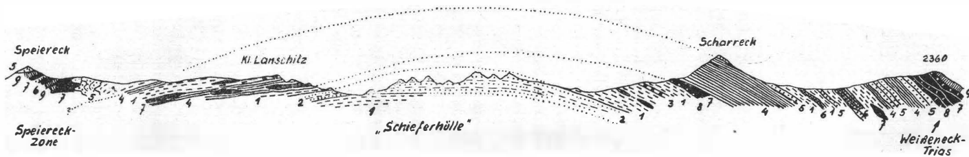
Fig. 27. Schematischer Schnitt über den Hauptkamm Speiereck-Scharreck. 1. Phyllite; 2. darin Quarzitschiefer; 3. Prasinit; 4. Kalkglimmerschiefer; 5. Quarzit und Quarzitschiefer (Typ Triasbasis); 6. Rauhwacke; 7. Dolomite; 8. Marmore; 9. Liasschiefer und Breccien, Schwarzeckbreccie (Jura-Kreide der Hochfeindentwicklung).
