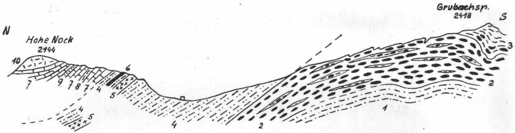
Fig. 3. Schnitt Grubachspitze—Hohe Nock. 1. Liasschiefer mit wenigen Lagen phyllitischer Breccie; 2. Schwarzeckbreccie mit besonders schieferreichen Linsen; 3. grüne Schiefer, zum Teil mit Geröleinstreung; 4. Glimmerschiefer- und Gneisdiaphthorite des Twenger Kristallins, darin 5. grober Granitgneis und 6. Aplit; 7. grauer Bändermarmor; 8. grüner Phyllit; 9. Serizitquarzit; 10. heller Dolomit.
