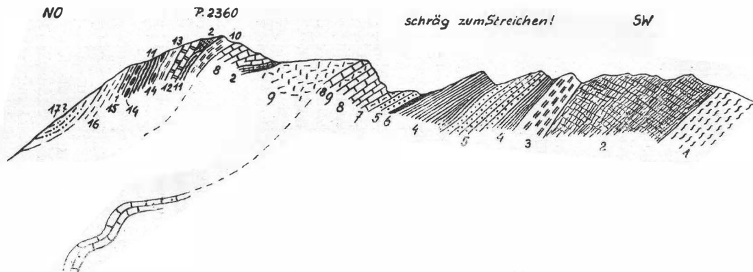
Fig. 26. P. 2360 im Hauptkamm zwischen Weißeneck und Scharreck. 1. Graue Phyllite; 2. gelbe Rauhwacken; 3. dunkle kalk-sandige Schiefer (Lias); 4. Kalkglimmerschiefer; 5. heller Quarzit und Quarzitschiefer; 6. Serizitschiefer; 7. heller Marmor; 8. grauer Bändermarmor; 9. heller Dolomit, weiter im Hang gebankt; 10. Liasschiefer mit Marmor, Dolomit und Schieferbreccienlagen; 11. grauer Quarzitschiefer (Bänderschiefer mit Radiolarit); 12. grauer Marmor bis Kalkglimmerschiefer; 13. sandig-kalkiger Phyllit; 14. typische Schwarzeckbreccie im engeren Sinne; 15. grüner Schiefer mit Geröllen; 16. grüner Phyllit (zu Schwarzeckbreccie); 17. Kristallin?
