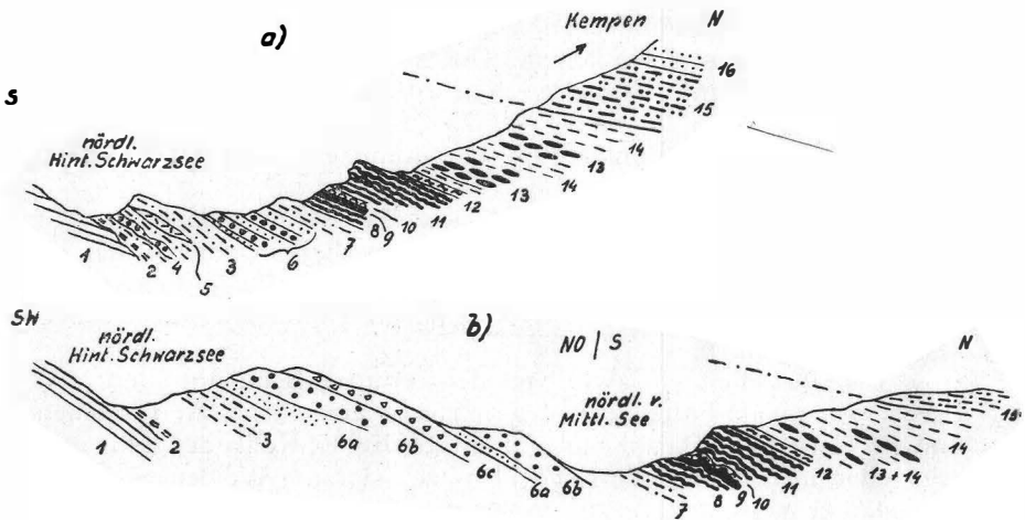
Fig. 10. Jura-Kreide im Schwarzseekessel. 1. Hauptdolomit mit braun verwitterter Oberfläche; 2. milder schwarzer Tonschiefer; 3. karbonatführende dunkle phyllitische Schiefer, zum Teil sandig; 4. schmale Lagen von phyllitdurchwirkter Dolomitbreccie (etwas Quarzit); 5. Linse von dunklem Dolomit; 6. Haupthorizont der Sandsteine und Breccien des Lias; 6a. karbonatischer Sandstein; 6b. vorwiegend reinere Dolomitbreccien; 6c. gröbere und quarzitreichere Breccien; 7. karbonatisch-sandiger phyllitischer Schiefer; 8. unterer Radiolarit; 9. Aptychenkalk mit 10. Breccienlage; 11. oberer Radiolarit, nach oben in grüne quarzitishe Schiefer übergehend; 12. grauer Bänderschiefer; 13. braune Dolomitbreccie mit Schollen grüner Schiefer (Schwarzeckbreccie im engeren Sinne); 14. grüne phyllitische Schiefer, vereinzelt mit Geröllen; 15. diaphthoritisches Twenger Kristallin; 16. Quarzite der Triasbasis.
