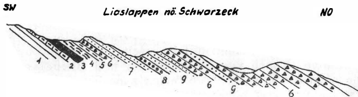
Fig. 9. 1. Hauptdolomit; 2. gelber Dolomit (»Eisdolomit«); 3. milder, schwarzer Tonschiefer, zu tiefst schmale phyllitische Dolomitbreccie; 4. feinlagiger dunkler Schiefer; 5. dunkler karbonatisch-sandiger Schiefer; 6. grobe, graugelbe Dolomitbreccie mit Quarzitschollen; 7. plattige Sandsteine, gleich Brecciengrundmasse und quarzreiche Feinbreccien; 8. braune quarzfreie Dolomitbreccie; 9. Sandsteine.
