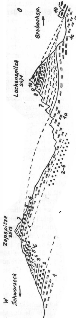
Fig. 14. 1. Liasschiefer, besonders graue Kalkschiefer; 1 a. mit Lagen von phyllitischer Breccie; 2. gelbliche Dolomitbreccie mit Quarzschollen; 3. grauer Phyllit; 4. Sandsteine und Feinbreccien; 5. hellgraue reine Dolomitbreccie; 6. ähnlich 2.; 7. harter dunkler bänderiger Phyllit; 8. phyllitreiche verschieferete Breccie; 9. grüner Schiefer; 10. Schwarzeckbreccie in engerem Sinne.
