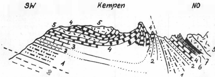
Fig. 2. Basale Trias der Lantschfeldecke am Kempfen-Himmelwand. 1. Twenger Kristallin; 2. heller Quarzit und Quarzitschiefer; 3. hellgrauer Marmor; 4. grauer Bändermarmor; 5. hellgrauer massiger Dolomit; 6. Rauhwacke; 7. dolomitische Quetschschiefer; 8. grüne Schiefer der Schwarzeckbreccie.
