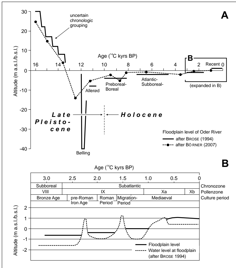
Fig. 3: Changes in the floodplain level of the lower Oder River. A: General development during the late Pleistocene and Holocene (after BROSE 1994, BÖRNER 2007, adapted). B: Detailed development during the late Holocene (after BROSE 1994, adapted). Abb. 3: Veränderungen des Auen-niveaus der unteren Oder. A: Generelle Entwicklung während des Spätpleistozäns und Holozäns (nach BROSE 1994, BÖRNER 2007, verändert). B: Detaillierte Entwicklung während des Spätholozäns (nach BROSE 1994, verändert).
