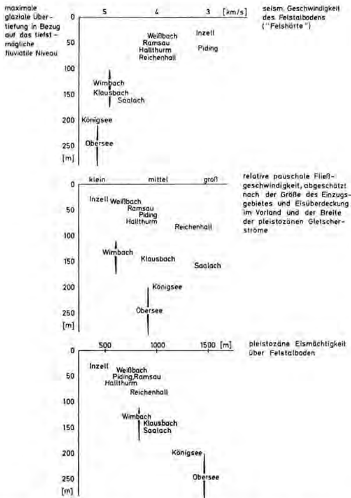
Abb. 6: Die glazialen Übertiefungen im Saalachglatschergebiet in Abhängigkeit a) von der Härte des Felsbettes, b) von der pauschalen Fließgeschwindigkeit der Eisströme und c) von der Eismächtigkeit im Pleistozän.
