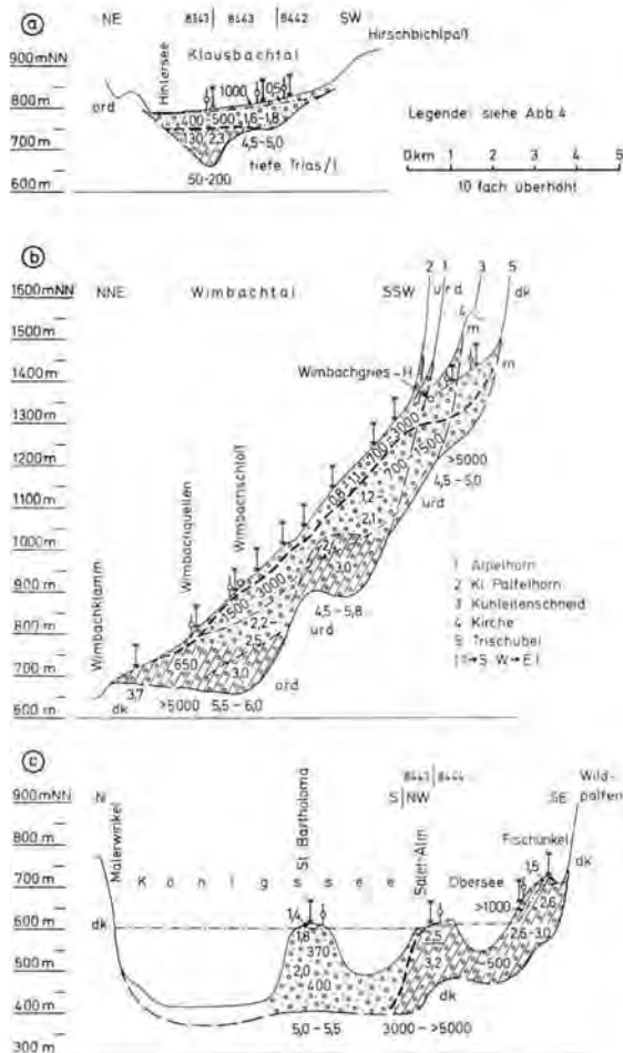
Abb. 5: Längsprofil durch das Klausbachtal, Wimbrachtal und das Königssee-Obersee-Becken mit Verteilung der gemessenen km/s- und Qm-Werte und der glaziogeologischen Interpretation.
