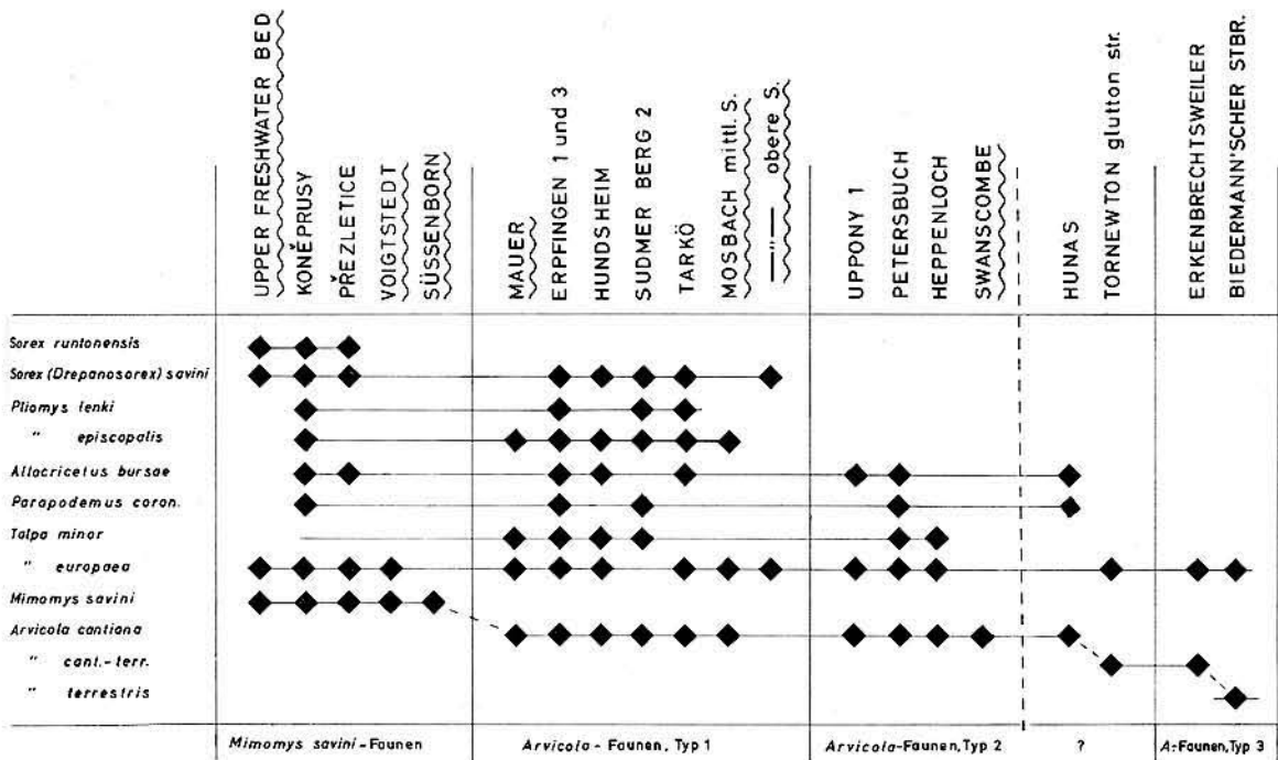
Abb. 1. Die zeitliche Verbreitung stratigraphisch wichtiger Kleinsäugerarten in europäischen Faunen des Pleistozäns. Fluviale Lagerstätten sind durch Wellenlinien gekennzeichnet, da sie meist ärmer an Kleinsäufern sind.
