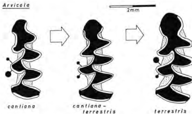
Abb. 2. Die Entwicklung der Schmelzbandverhältnisse bei den Arvicola -Formen in Mitteleuropa. Arvicola cantiana (Elster-Riß), Arvicola cant. terr. Übergangsform (Riß-Eem); Arvicola terrestris (Eem-Holozän).
