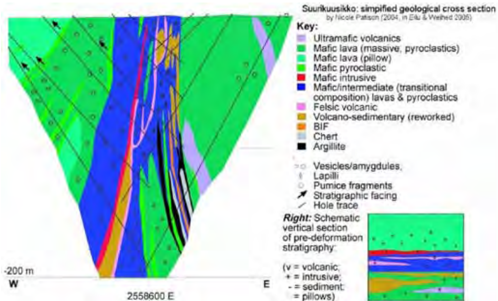
Figure 17: Simplified geological cross section of the Suurikuusikko Trend (EILU & WEIHED, 2005).
