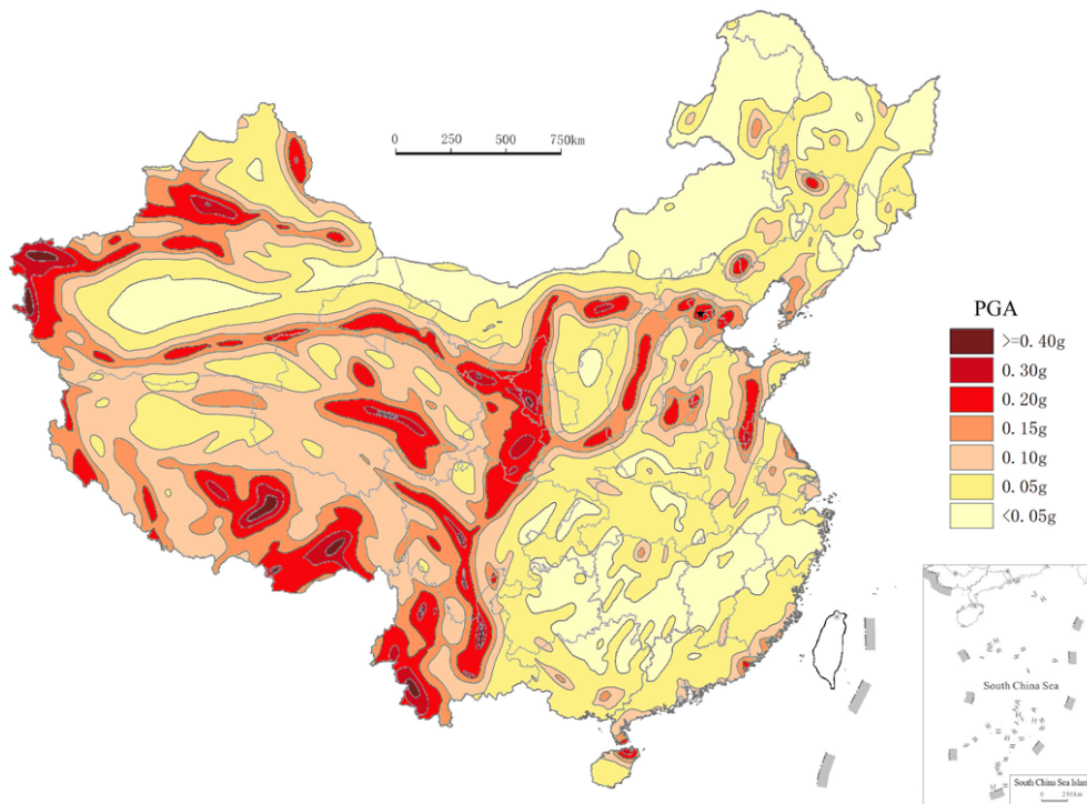
Fig. 2. Seismic ground motion parameter zonation map of China.
