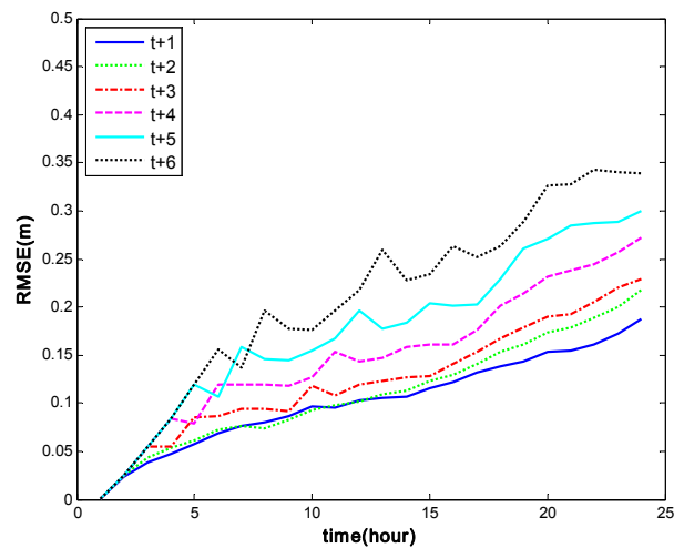
(b) R-NARX
