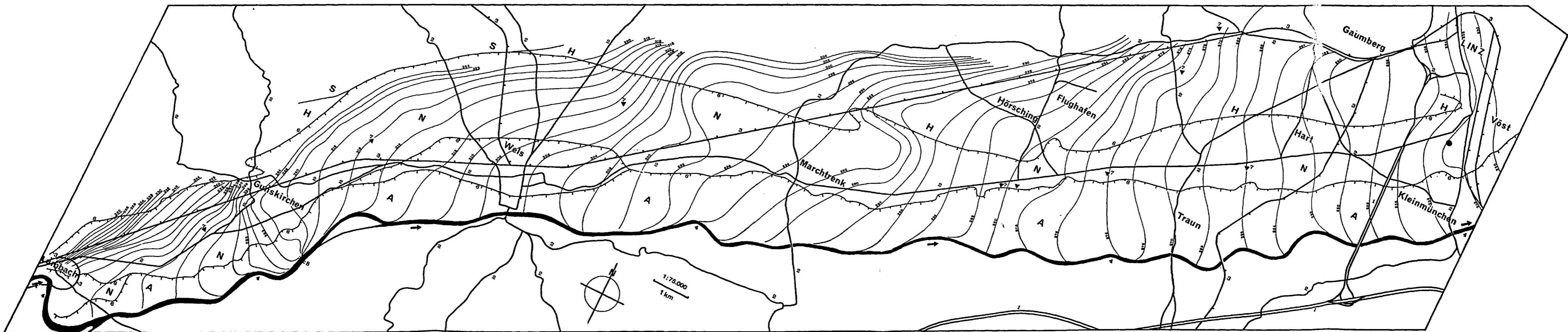
Abb. 6: Grundwasserschichtenplan der Welsener Heide, aufgenommen vom Hydrografischen Dienst des Amtes der öö. Landesregierung vom 3. — 5. 11. 1964 bei Niedrigwasser (NW).
