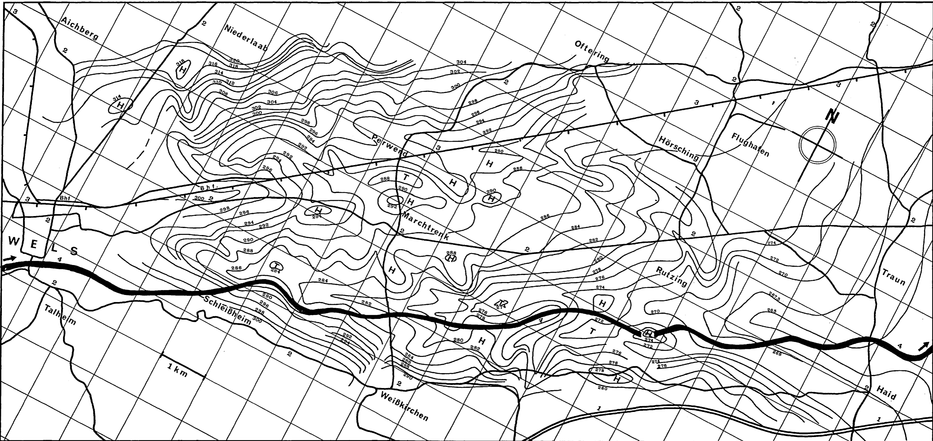
Abb. 8: Schlierrelief der Welser Heide, von D. KOMPOSCH, Hydrografischer Dienst.
