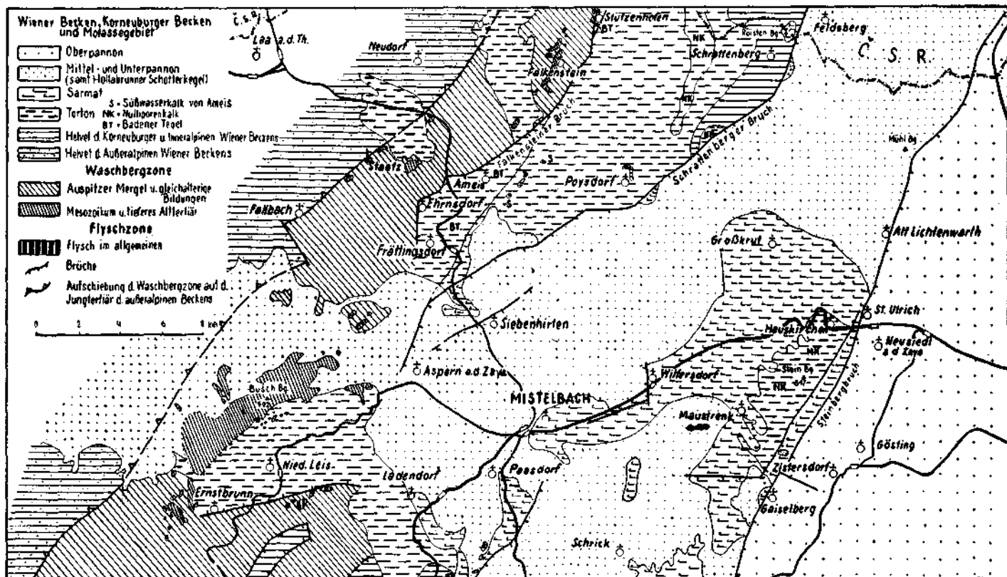
Abb. 1. Abgedeckte geologische Kartenskizze des nördlichen Inneralpinen Wiener Beckens im Bereich von Poysdorf—Mistelbach—Zistersdorf.
