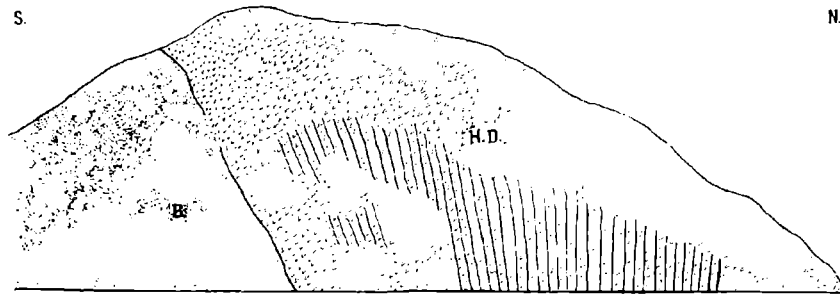
Aufschluß im Norden des Neokombrechtes an der Waldmühle.
