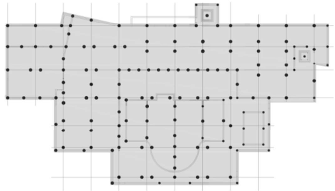
Abb. 9: Bewehrungsummantelung und Gründungsplatte mit Pfählen (DI Nessler, 2009)
