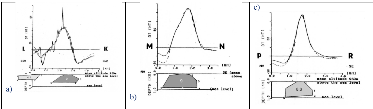
Abb. 2.34: Modellrechnungen Liebenau nach HEINZ, (1992)
