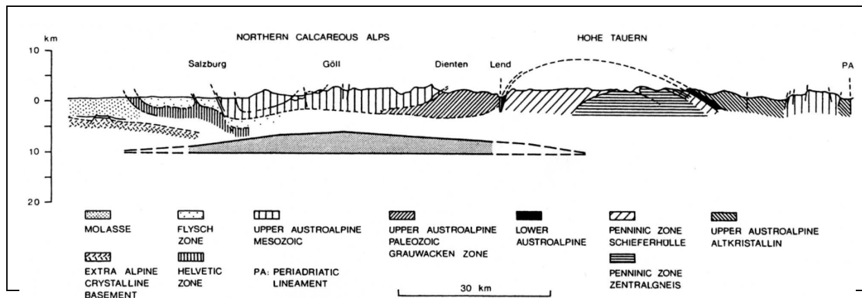
Abb. 2.7.: Geologische Profil durch die Ostalpen mit dem von BLEIL & POHL (1976) berechneten Störkörper der Berchtesgadener Anomalie.
