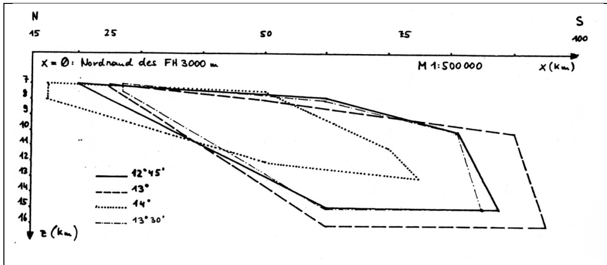
Abb. 2.13: Darstellung des Modellkörpers „Böhmische Masse“ anhand mehrerer Profile, nach REISNER (1988), \kappa=38 \times 10^{-3} (SI).
