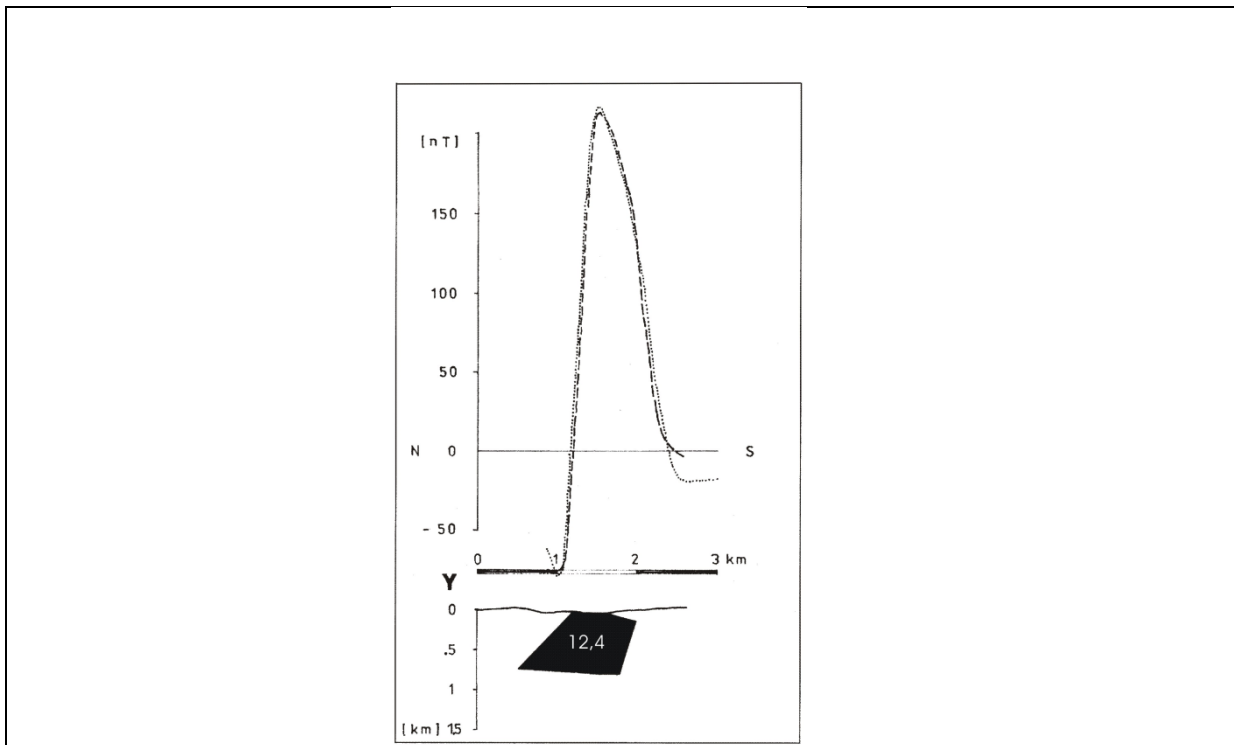
Abb. 2.29: Modellierung der Anomalie von Sandl (GNOJEK & PŘICHYSTAL, 1997), die Suszeptibilität ist mit 12,4 \times 10^{-3} (SI) angenommen worden.
