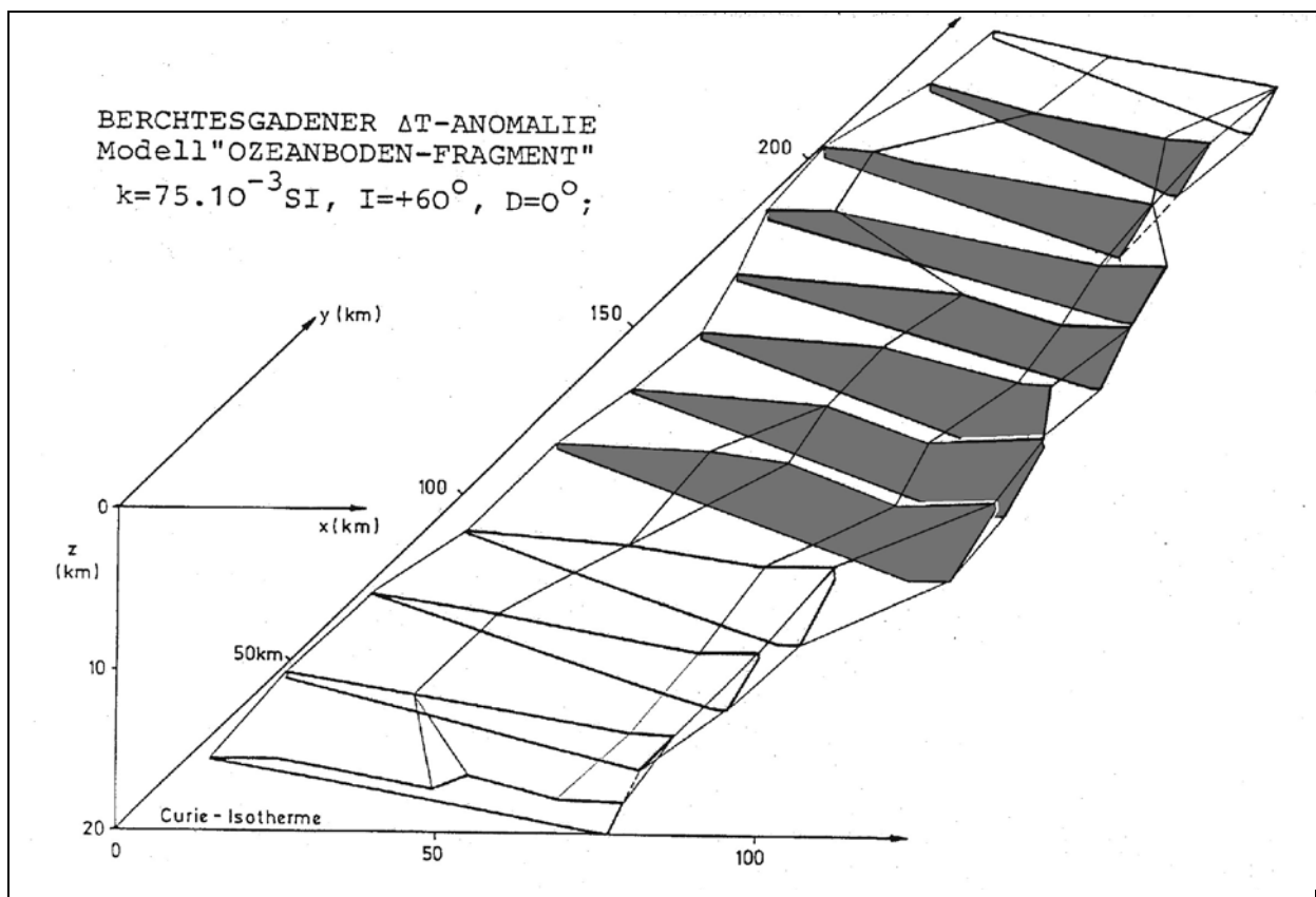
Abb. 2.11: N-S Schnitte durch den errechneten Störkörper nach REISNER (1988). Die in der Abb. 2.3 eingetragenen Profile sind grau dargestellt.
