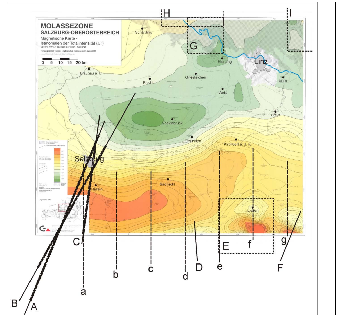
Abb. 2.3: Darstellung der Anomalien der magnetischen Totalintensität \Delta T (nach MOTSCHKA et al., 2006) und die Lagen der Profile der 2D Modellrechnungen (durchgezogene [A, B, C, D und F] und strichlierte Linien [a bis g] sowie der Bereiche der 3D Modellrechnungen [gepunktete Linien, E, G, H, und I]). Bei den Profilen A) (BLEIL & POHL, 1976), B) (PUCHER & HAHN, 1979) und C) (HÜBL, 1991) sind sowohl die Lage des berechneten Profilschnitts (dünnere Linie), als auch die Lage des Profils des Modellkörpers (dickere strichlierte Linie) eingetragen.
