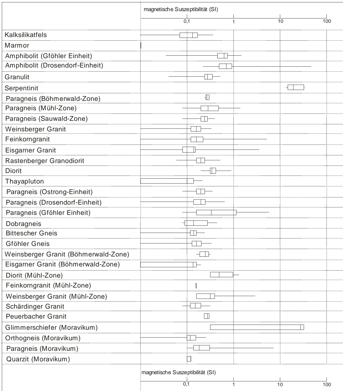
Abb. 2.24: graphische Darstellung der statistischen Verteilungen von Tab. 2.2. Die Boxen erstrecken sich zwischen unterem und oberem Quartilwert, der Strich darin ist der Medianwert, der Mittelwert wurde nicht dargestellt.
