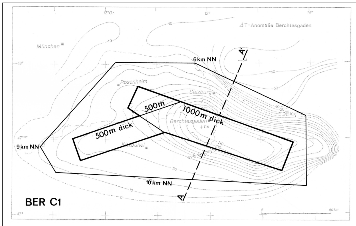
Abb. 2.8: Modell von PUCHER & HAHN (1979), die Profillinie AA' entspricht dem Profil B in Abb. 2.3.
