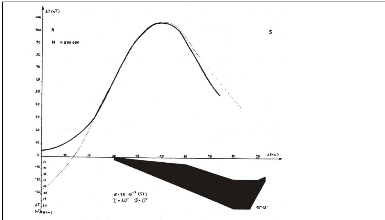
Abb. 2.12: Modell für das Profil 13°15' nach REISNER (1988): gemessene Werte (punktirierte Linie) gegenübergestellt den berechneten Werten (dickere durchgezogene Linie).
