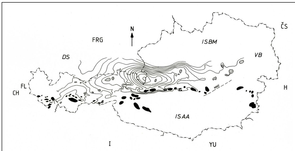
Abb. 2.20: Lage der in den tektonischen Modellen von H. HEINZ als vermutetes Südpenninikum eingestuft Anomalien HEINZ & HÜBL, 1988).
