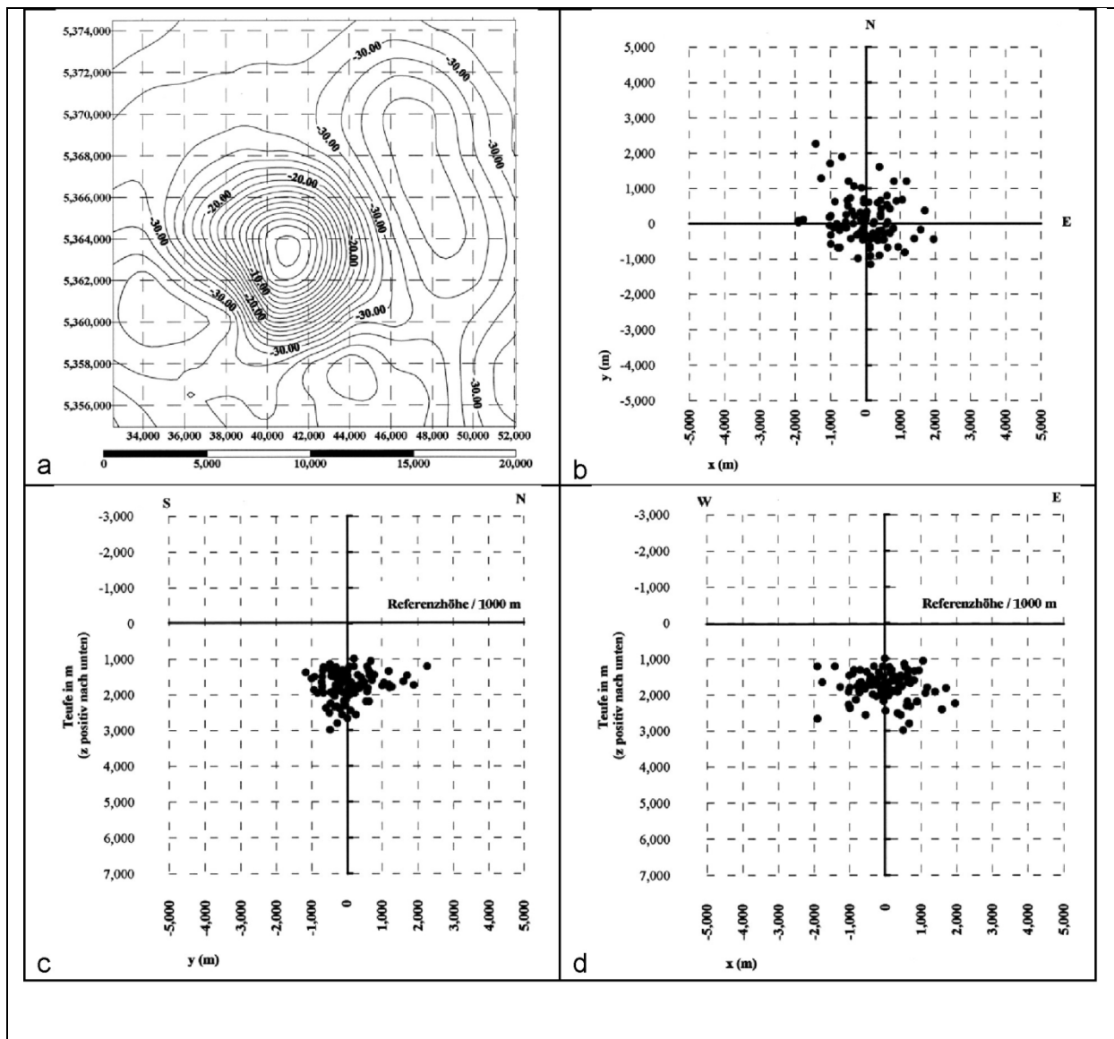
Abb. 2.26: Ergebnisse der magnetischen Modellierung durch R. ARNDT. a) Lage der Anomalie (B in Abb. 2.23) b) Lage der Tiefenpunkte im Horizontalschnitt c) Lage der Tiefenpunkte im NS Profil d) Lage der Tiefenpunkte im EW Profil. Die Referenzhöhe ist die Höhe des Flughorizonts.
