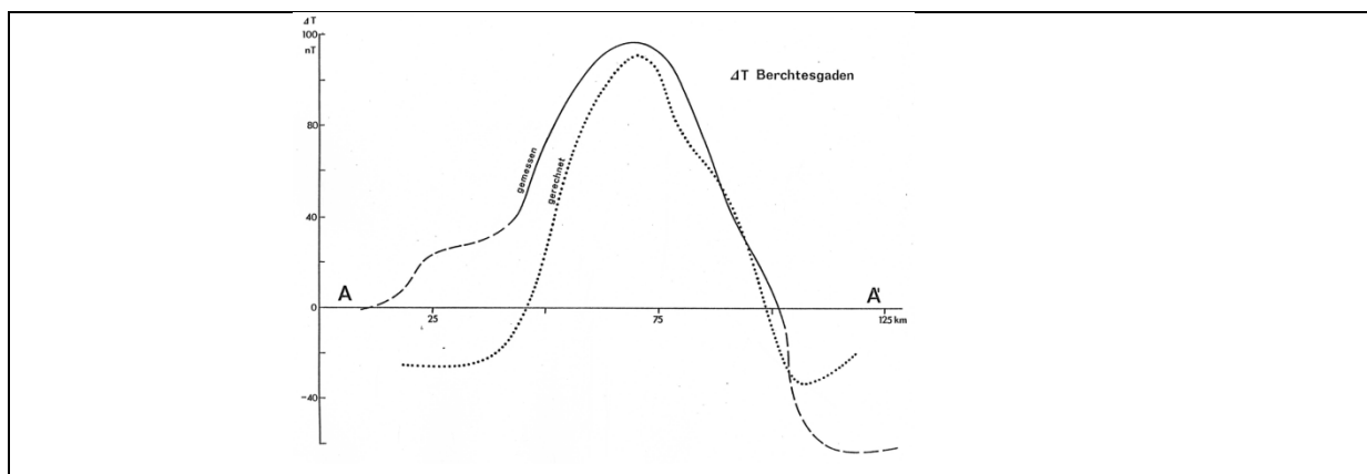
Abb. 2.9.: Unterschied zwischen gemessener und berechneter magnetischer Totalintensität ( \Delta T ) im Profil von Abb. 2.8.
