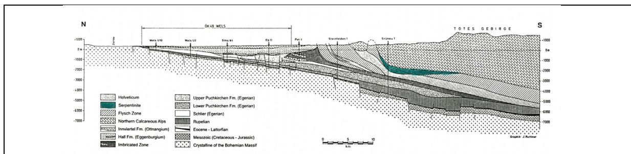
Abb. 2.4: Profil durch die Molassezone Oberösterreichs und deren Untergrund im Abschnitt Wels mit der Lage einzelner Bohrungen (WAGNER, 1996). Die Serpentine an der tektonischen Basis der Nördlichen Kalkalpen in der Bohrung Grünau 1 sind blaugrün hervorgehoben.
