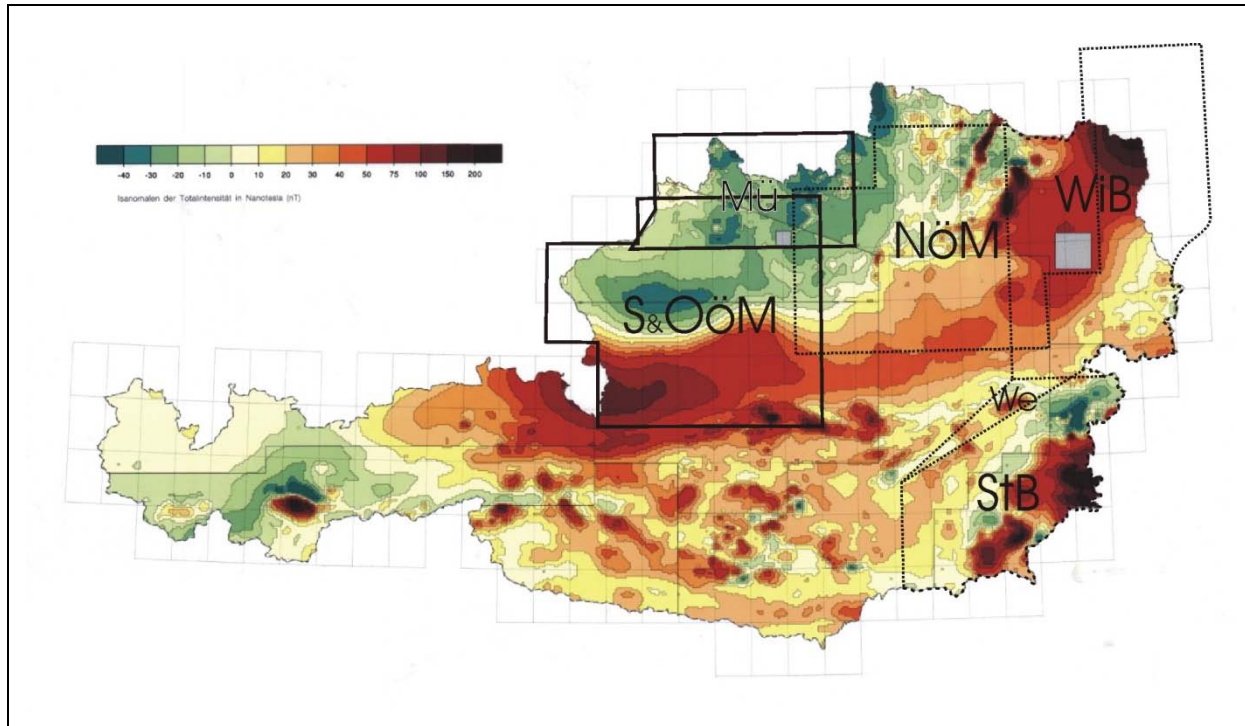
Abb. 1: stark verkleinerte Darstellung der aeromagnetischen Karte von Österreich 1 : 1.000.000 (SEIBERL, 1991). Durchgehend umrandet: die hier behandelten Untersuchungsgebiete „Molassezone Salzburg und Oberösterreich“ (S&OöM) und „Mühlviertel“ (Mü), strichliert umrandet: die früher bearbeiteten Untersuchungsgebiete „Molassezone Niederösterreichs und angrenzende Gebiete“ (NöM) (SEIBERL et al., 2002), „Wiener Becken und angrenzende Gebiete“ (WiB), „Wechsel“ (We), sowie „Steirisches Becken und Südburgenländische Schwelle“ (StB) (BIEBER et al., 2004).
