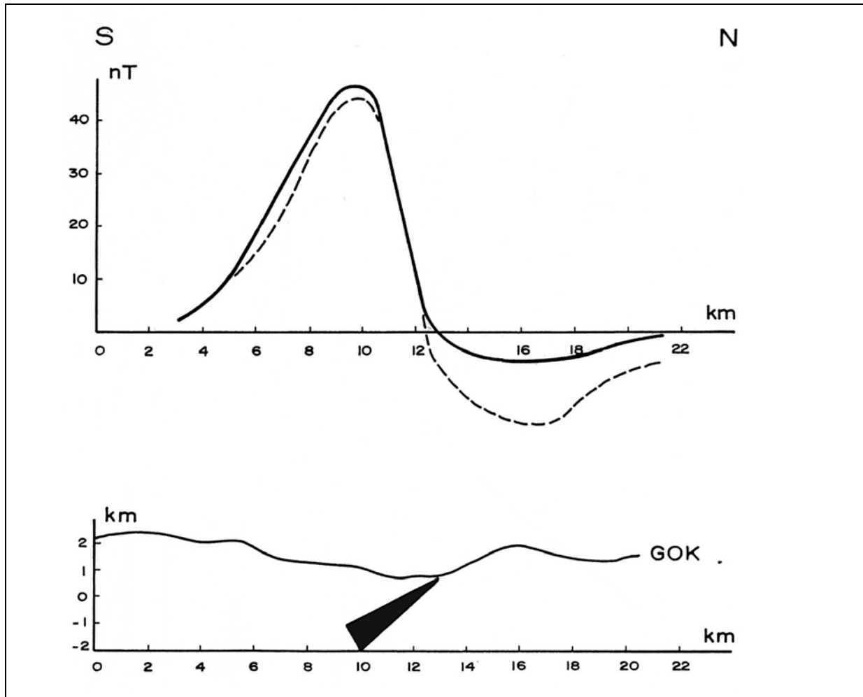
Abb. 2.16: Modell Haus im Ennstal: nach HEINZ et al. (1987): Profil D in Abb. 2.3, die angenommene Suszeptibilität \kappa = 7 \times 10^{-3} SI.
