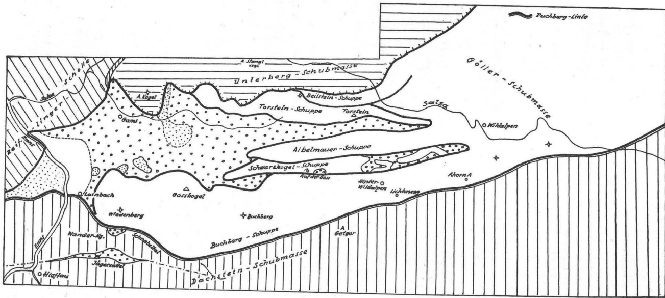
Abb. 4. Die Aufsplitterung der Gölleschubmasse in einzelne Schuppen.
