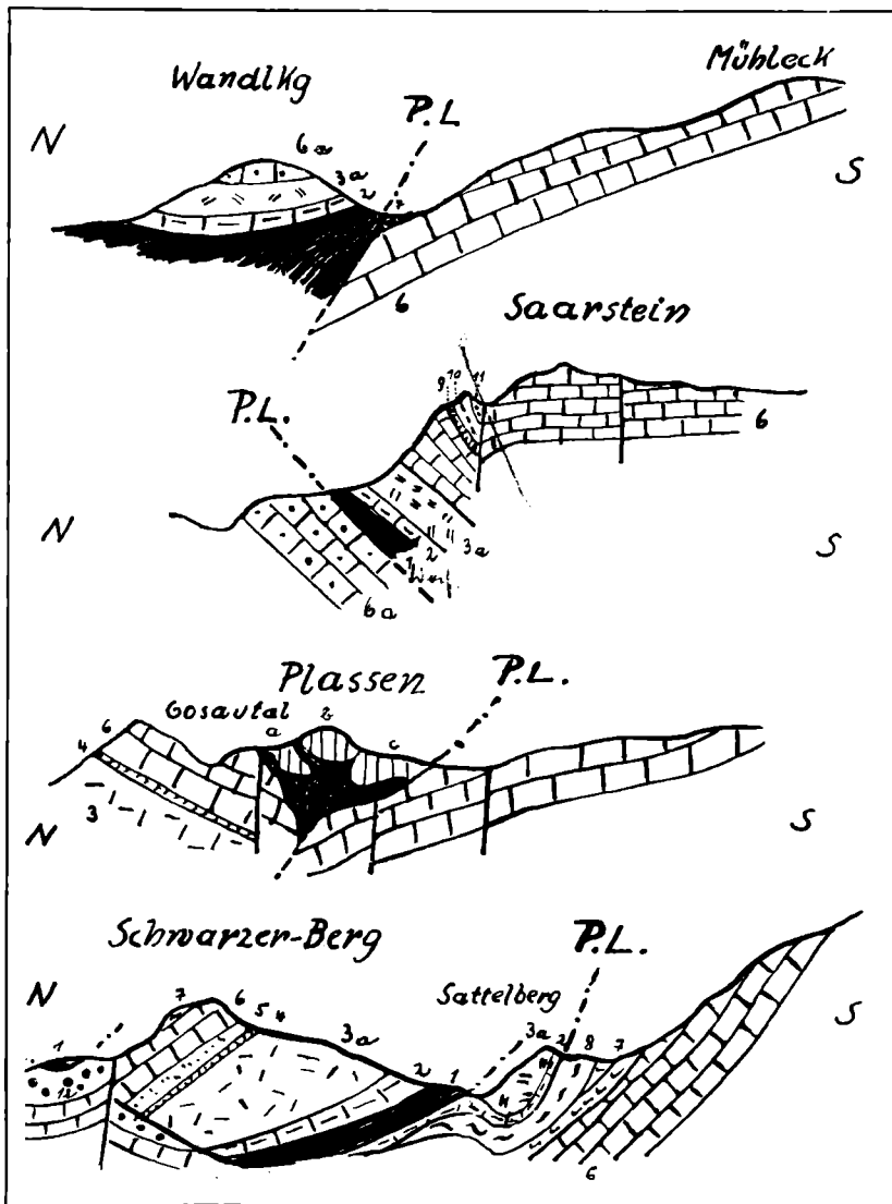
Abb. 8 (nach Geyer, Medwenitsch, Ampferer, Plochinger). 1 Werfener Schichten; 2 Gutensteiner Kalk bzw. Dolomit; 3 Wettersteinkalk; 3a Ramsaudolomit; 4 Raiblerschichten; 5 Hauptdolomit; 6 Dachsteinkalk; 6a Hallstätter Kalk; 7 Liaskalk; 8 Strubbergsschichten; 9 Hornsteinschichten; 10 Oberalmschichten; 11 oberster Malmkalk; 12 Schrambach- und Roßfeldschichten. a, b, c Schollen aus mesozoischen Schichten am Plassen (juvavisch). P. L. Puchberglinie.
