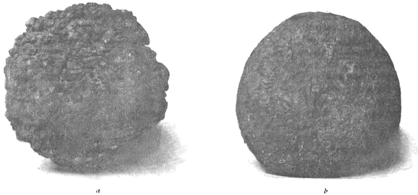
Eozängerrolle von Radstadt im Pongau.
