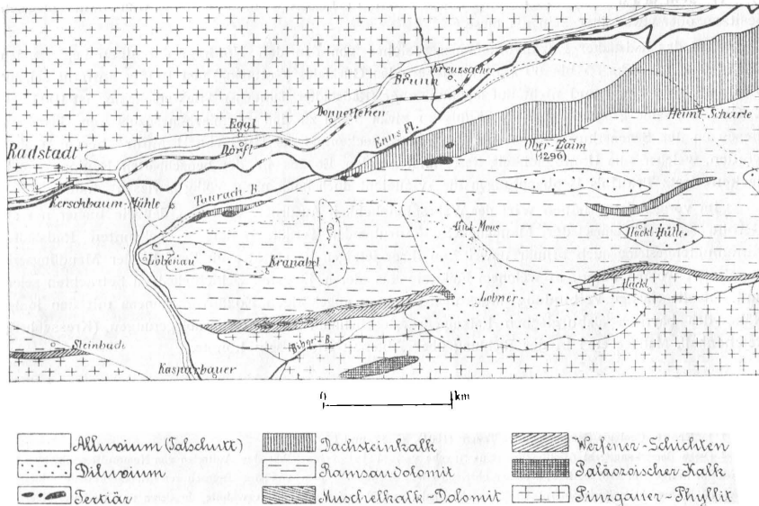
Geologisches Kärtchen der Mandlingkette östlich von Radstadt, aufgenommen von F. Trauth.
