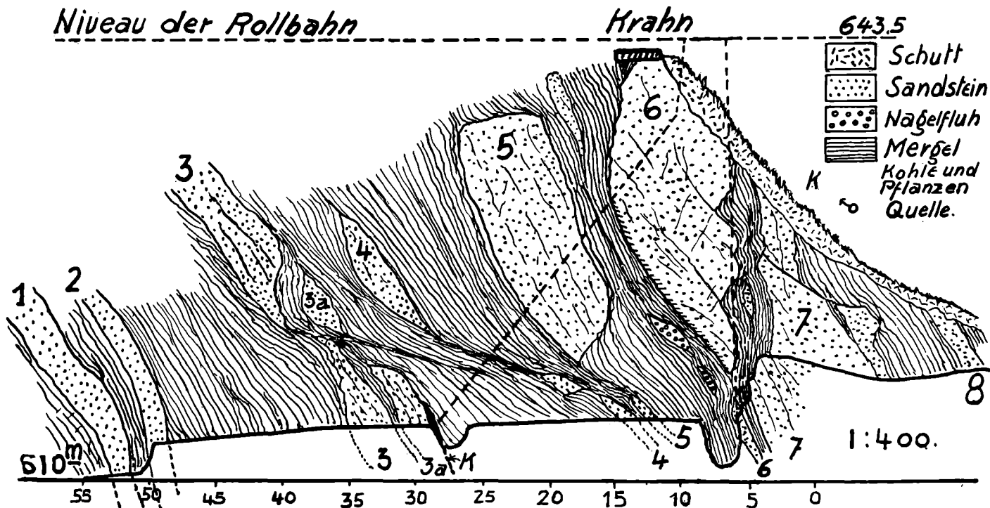
Fig. 6. Profilsicht des rechten Hanges der Baugrube für den Staudamm im Rempen. Gequetschte und gestreckte Molasseschichten (Aquitane). Nach den Vermessungen von Ing. DUBS, ergänzt von H. SCHARDT.
