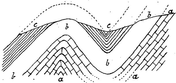
Abb. 1. Gewöhnliche Falte.
