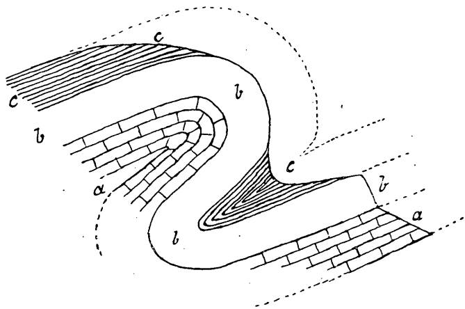
Abb. 2. Liegende Falte.
