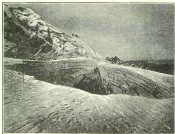
Fig. 6. Einsturz der Oberfläche des Gletschers von Tête Rousse.
