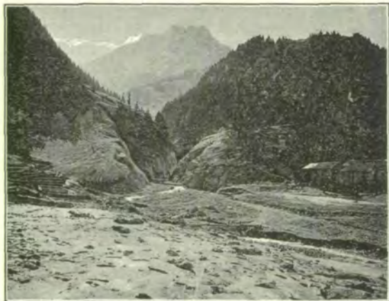
Fig. 8. Ausgang der Schlucht bei Bionnay.
