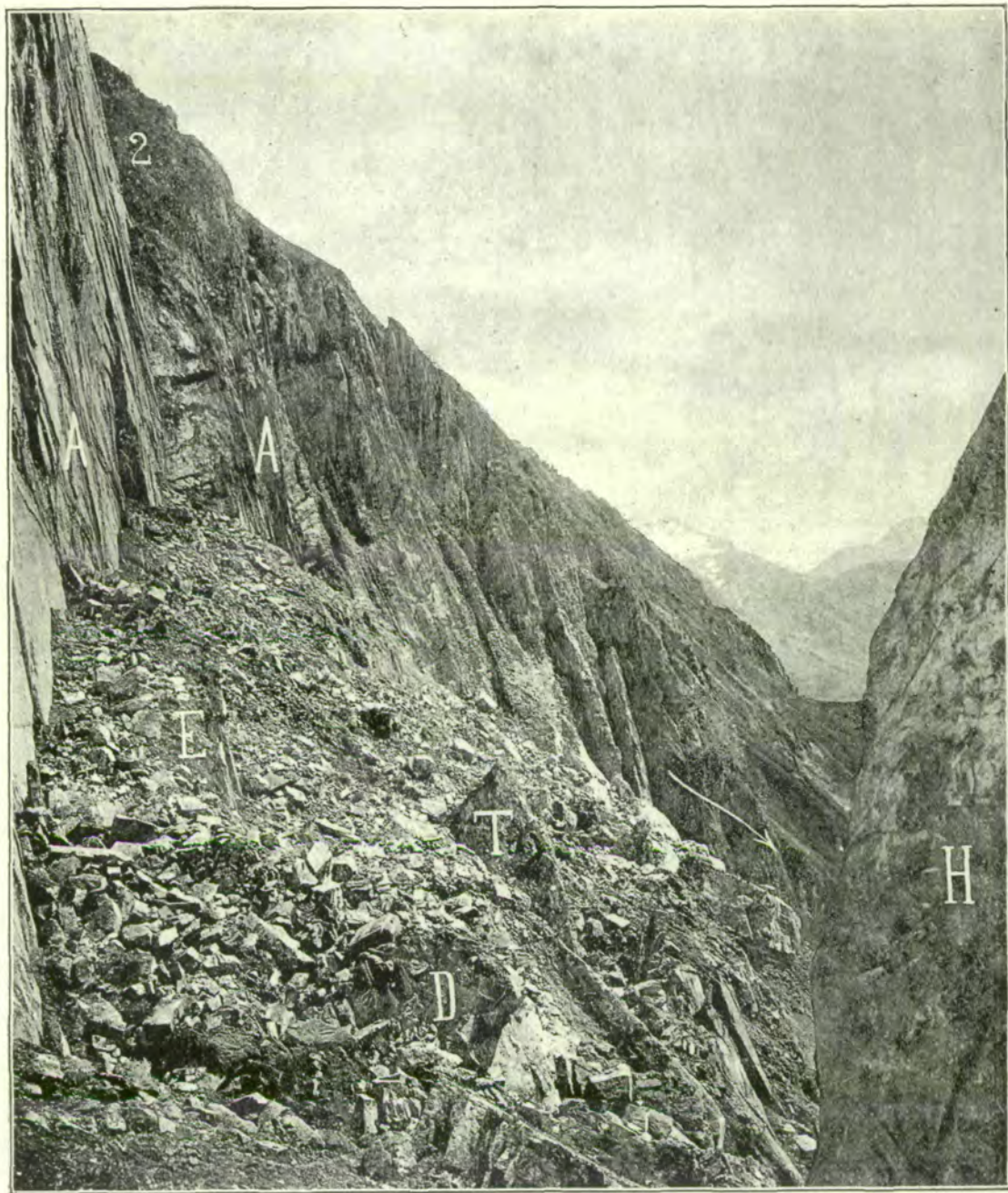
Nach Ob.-Ing. V. Pollack's Aufnahme. (Aus dem Jahrb. d. k. k. geol.-R.-Anst. 1892, Fig. 2, Taf. XVII.)
