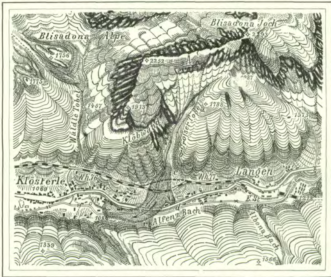
Nach einer Skizze des Herrn Ob.-Ing. V. Pollack. (Aus dem Jahrb. d. k. k. geol. R.-Anst. 1892, S. 662.) Massstab 1 : 25.000.
