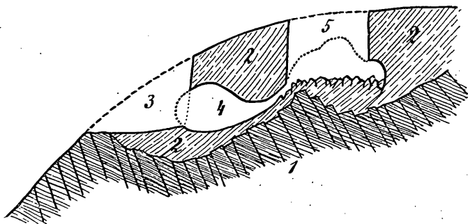
Fig. 5. Profil des Gletschers.
