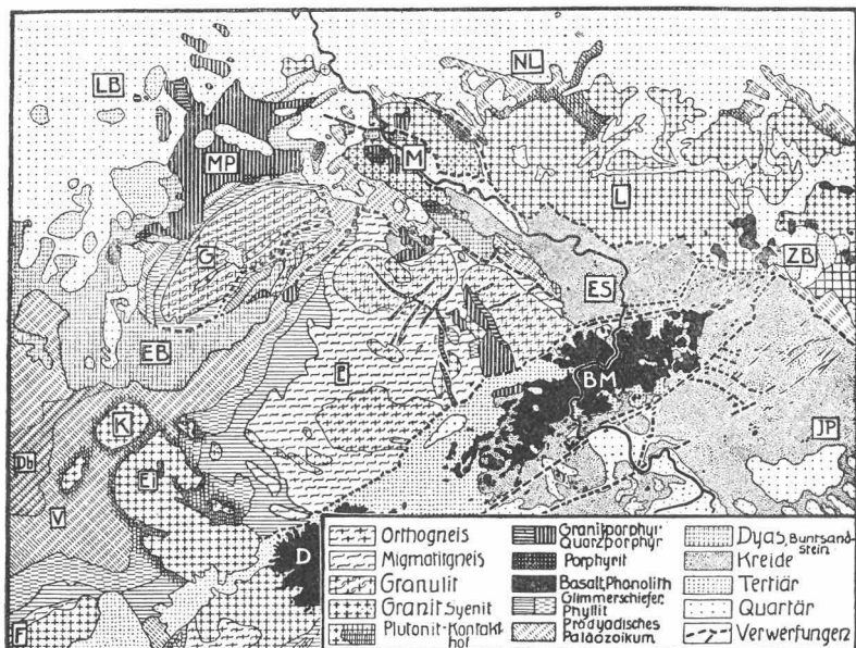
Fig. 3. Gesteinskundliche Übersicht Sachsens.
