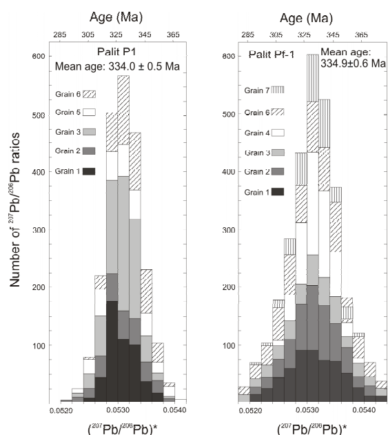
Abb. 2. Einzelzirkondatierungen nach der Evaporationsmethode an zwei Palitproben.
