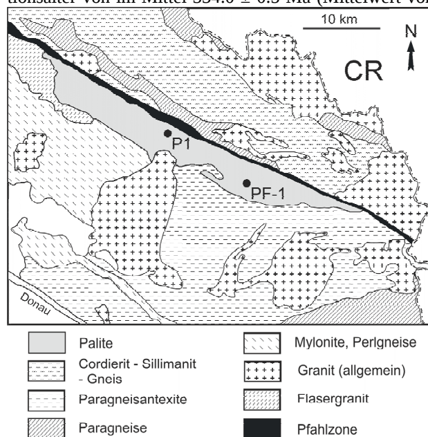
Abb. 1. Geologische Karte des Bayerischen Waldes.
