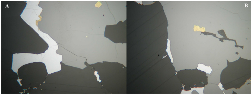
Abb. 8: Anschliff-Bilder der Bleiglanz-Zinkblende-Vererzung von Winkl . A: (// Pol) Zinkblende (hellgrau) mit Pyrit-Einschluss (hellgelb) und randlich an der Korngrenze zu Bleiglanz (weiß) auftretendem Pyrit, sowie Bleiglanz-Einschluss im Karbonat, (Vergr. 50 x). B: (// Pol) Zinkblende (hellgrau) mit Pyrit-(hellgelb) und Karbonat-(grau) Einschlüssen sowie mit randlich auftretendem Bleiglanz (weiß).
