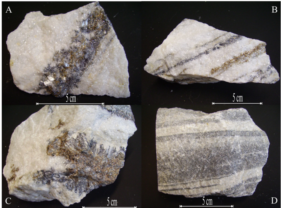
Abb. 7: Handstücke von im Westteil des Steinbruchs Winkl vorkommenden Marmoren. A, B: Mit brauner Zinkblende und grauem Bleiglanz lagenförmig vererzter weißer Dolomit-Marmor; C: Massige Bleiglanz-Zinkblende-Vererzung im Dolomit-Marmor; D: Unvererzter Bändermarmor.
