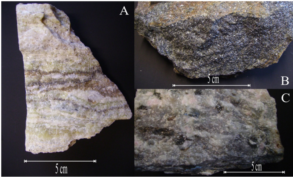
Abb. 3: Handstücke von im Steinbruch Kochholz vorkommenden Gesteinen. A: Braune Zinkblende-Lagen im Silikatmarmor; B: Massiger Amphibolit, C: Helles syenitisches Ganggestein mit dunklen Amphibolen.
