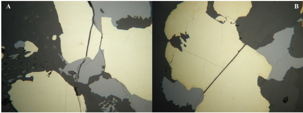
Abb. 6: Anschliff-Bilder der Pyrit-Zinkblende-Vererzung von Lichtenau. A: (// Pol) Hypidiomorphe Pyrit-Körner (hellgelb) und xenomorphe Zinkblende-Körner (hellgrau) in Karbonat-Matrix, gemeinsam tektonisch zerbrochen, (Vergr. 25 x). B: (// Pol) Tektonisch zerbrochener Pyrit (hellgelb) mit randlich auftretender Zinkblende (hellgrau), (Vergr. 25 x).
