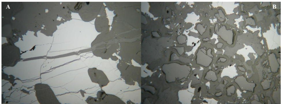
Abb. 4: Anschliff-Bilder der Zinkblende-Vererzung von Kochholz. A: (// Pol) Tektonisch zerbrochene, xenomorphe Zinkblende-Aggregate (hellgrau) mit Calcit verheilt in Karbonat-Matrix, (Vergr: 50 x). B: (// Pol) Feinkörnige xenomorphe Zinkblendes (hellgrau) zwischen serpentinisierten Silikatkörnern (grau) in Karbonat-Matrix (dunkelgrau), (Vergr: 25 x).
