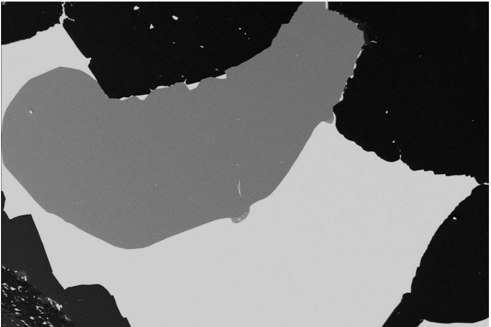
Abb. 9: REM-Aufnahme eines Zinnkies-Einschlusses (siehe Bildmitte) an der Korngrenze zwischen Zinkblende und Bleiglanz, aus der Vererzung im weißen Dolomit-Marmor von Winkl, (Vergr. 150 x).
