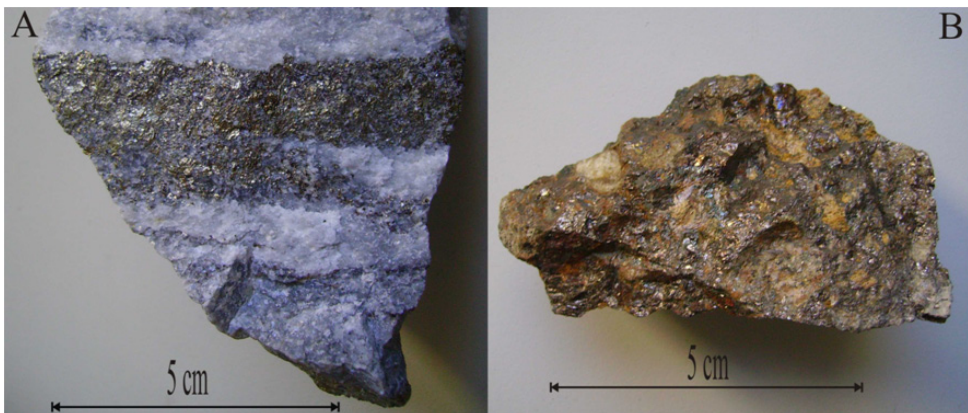
Abb. 5: Handstücke von im Steinbruch Lichtenau vorkommenden vererzten Gesteinen. A: Pyrit-Zinkblende-Lagen im Tremolit-Marmor, B: Massiger von Karbonaten durchsetzter Pyrrhotin.
