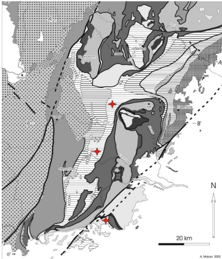
Abb. 1: Tektonische Übersicht über das Waldviertel, modifiziert nach MATURA (2003). Die Sterne verzeichnen die Fundpunkte Kochholz (südlich), Lichtenau (mittig), Winkl (nördlich). Die Legende ist der Abb. 2 zu entnehmen.
