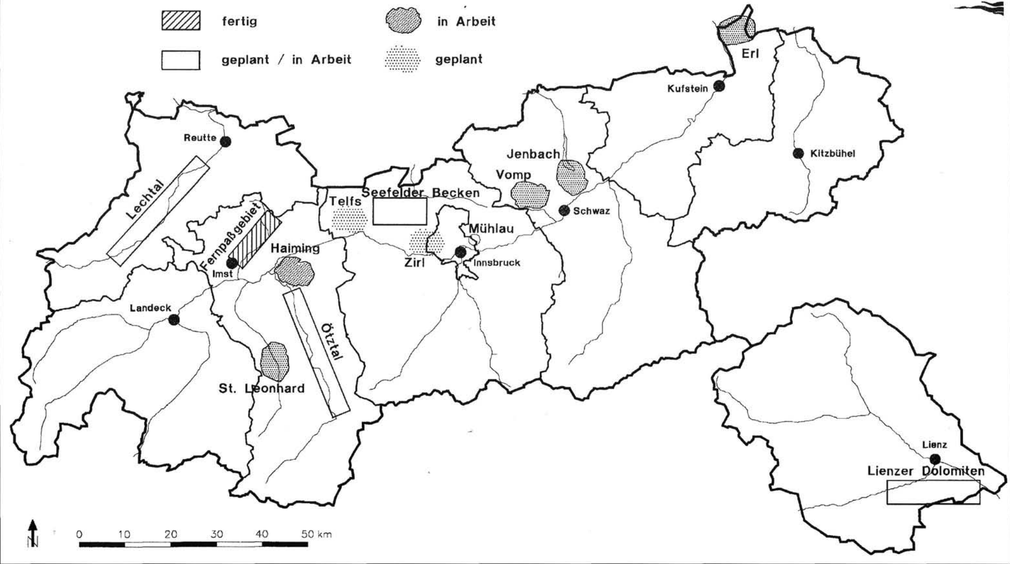
Abb. 3. Lage der Großquellenhydrogeologie- und Großraumgeologieprojekte.
