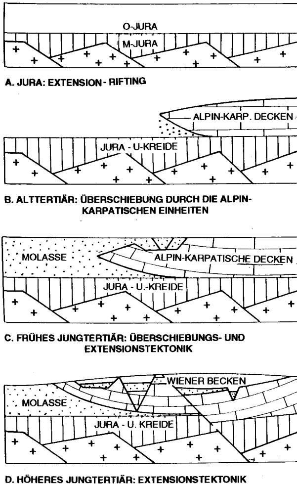
Abb. 11: Die einzelnen Entwicklungsstufen des Wiener Beckens (nach: W. LADWEIN et al., 1991).
