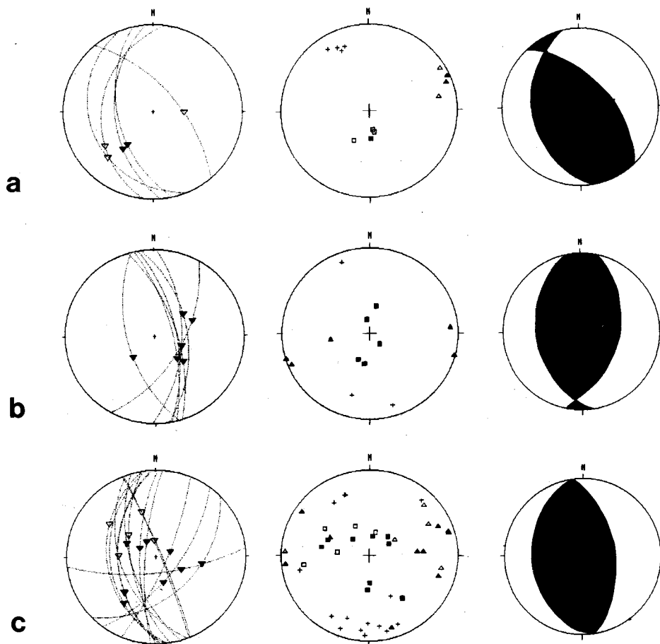
Abb. 8: E-W-Extension ab dem Baden: An den vorwiegend N-S-streichenden Flächen kommt es nur noch zu abschiebenden Bewegungen; (a) Mödling; (b) Wöllersdorf; (c) Mannersdorf.
