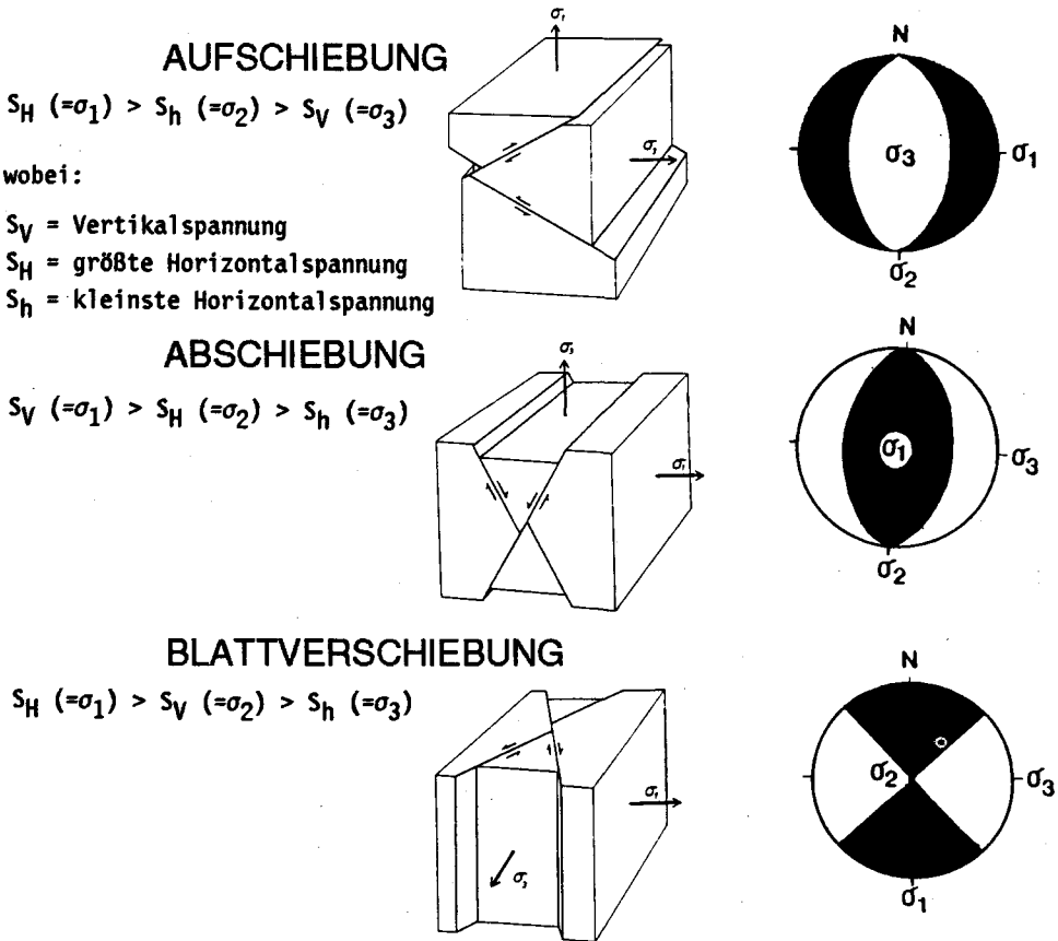
Abb. 5: Die drei Typen von Störungen nach E. ANDERSON (1951) und Darstellung der verursachenden Streßregime auf der unteren Halbkugel des Schmidt'schen Netzes (schwarz=Kompression; weiß=Extension).
