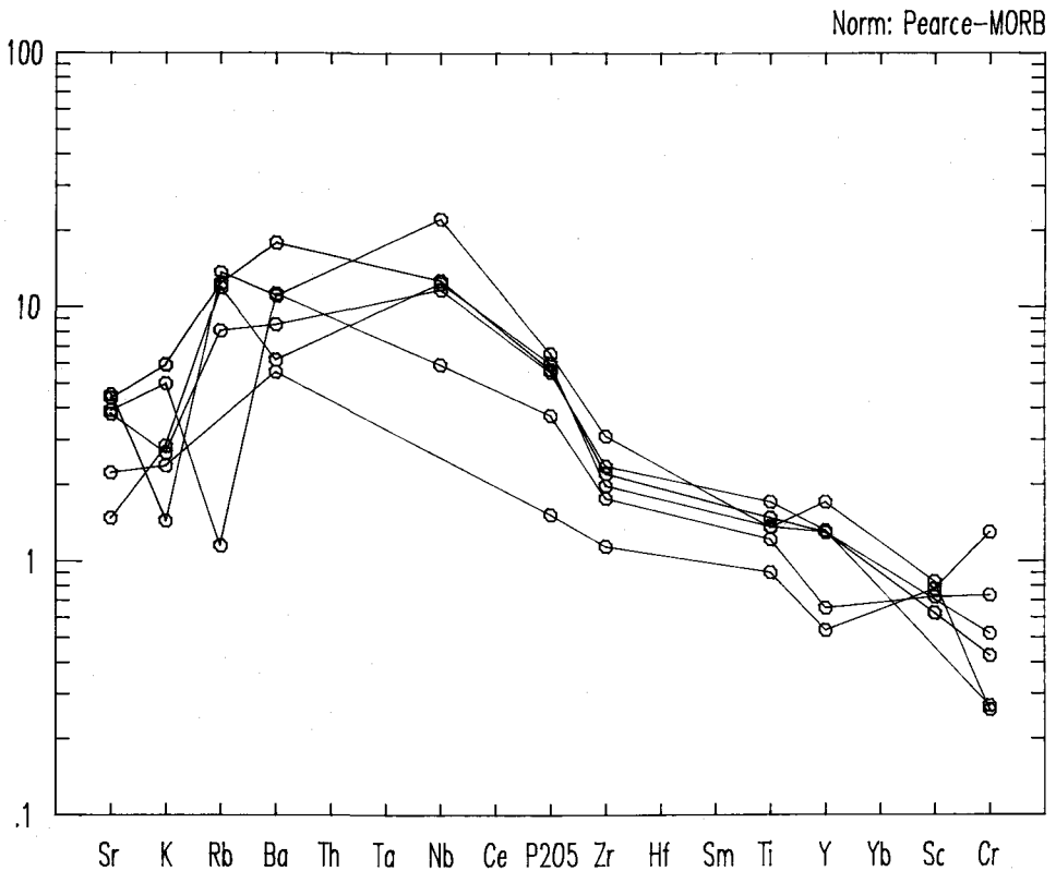
Multiementdiagramm normiert gegen MORB nach PEARCE (1982): Abb. 11: a) Darstellung der Vulkanite aus der Gosau von der Lokalität Eichberg; ● basaltische Zusammensetzungen.
