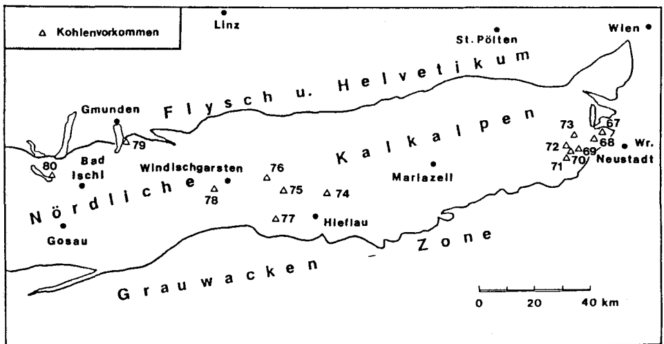
Abb. 7: Untersuchte Gosau-Kohlenvorkommen (Zahlen beziehen sich auf Tab. 8).
