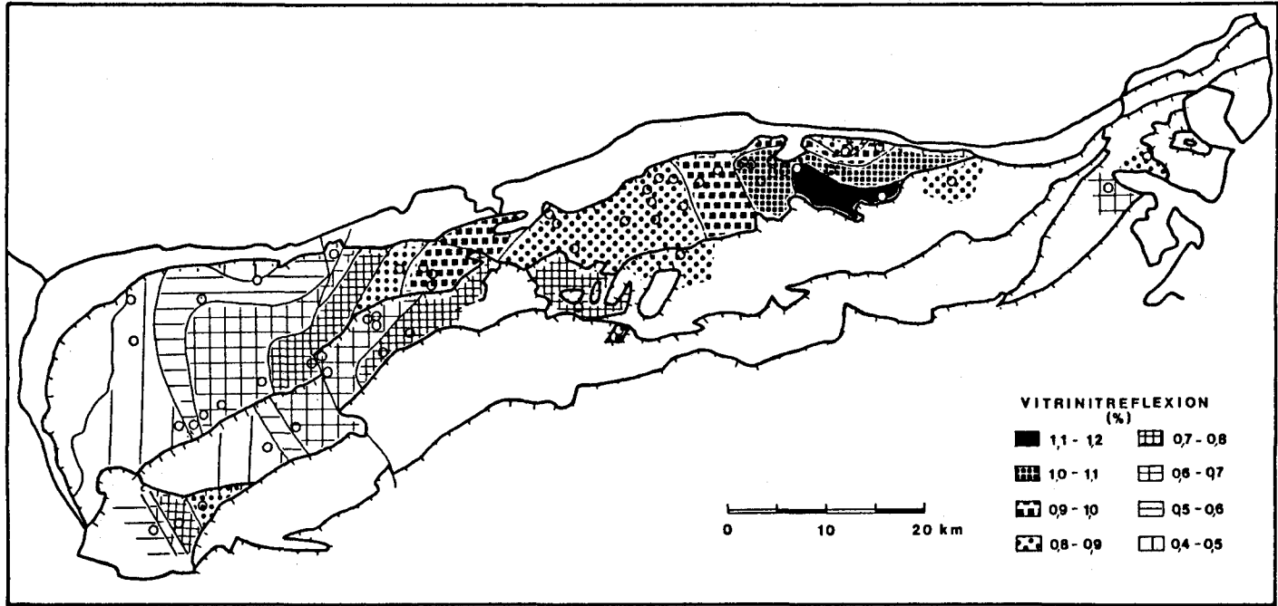
Abb. 3: Inkohlungskarte der Lunzer Schichten der östlichen Kalkvoralpen (Basis: Vitrinitreflexion).
