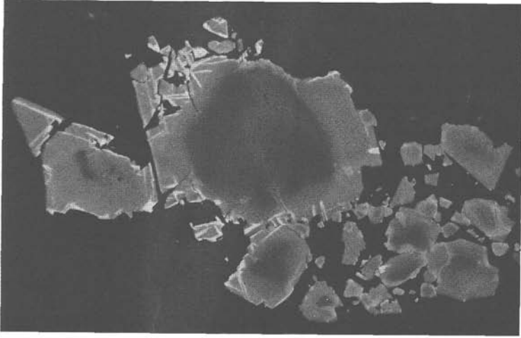
Abb. 25: Fuchs in Gstanach, Voralu (Steiermark). Chromit (dunkelgrau) in Granat (schwarz) zeigt randliche Umbildungs- bzw. Verdrängungssäume von Magnetit (mittelgrau), der seinerseits nach {111} Verdrängung durch Eisenglanz (lichtgrau), „Martitisierung“, aufweist. Anschliff, Ölimmersion, Vergr.: 500×
