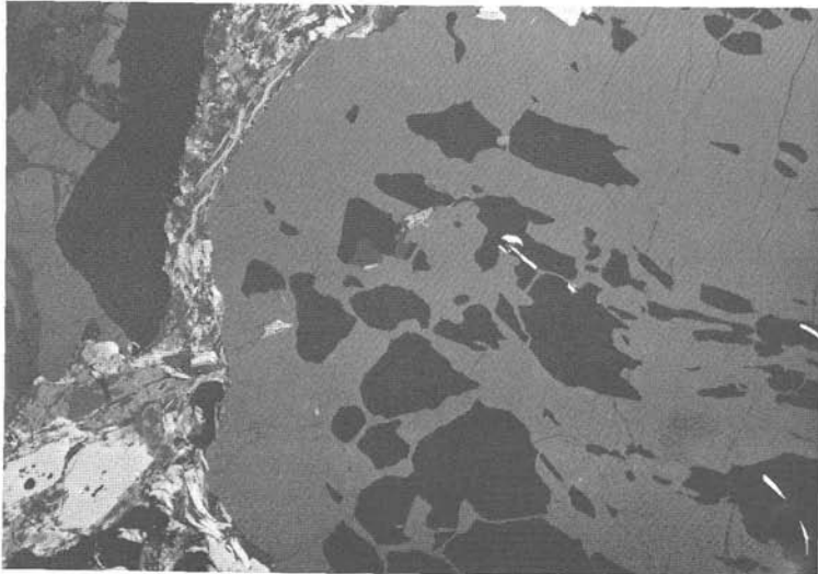
Abb. 24: Fuchs in Gstanach, Voralpe (Steiermark). Granat-Porphyroblast (mittelgrau) mit reichlich Einschlußzügen („sif“) bzw. Verdrängungsresten von Quarz (dunkelgrau), wenig Siderit (licht dunkelgrau) und kleinsten Graphit-Täfelchen (lichtgrau, fast weiß bis licht dunkelgrau – Reflexionspleochroismus!) weist randlich reichlich Graphit (linke Bildhälfte!), darin auch idiomorpher Ilmenit (hellgrau; linke, untere Bildecke), auf. Anschliff, Vergr.: 75×
