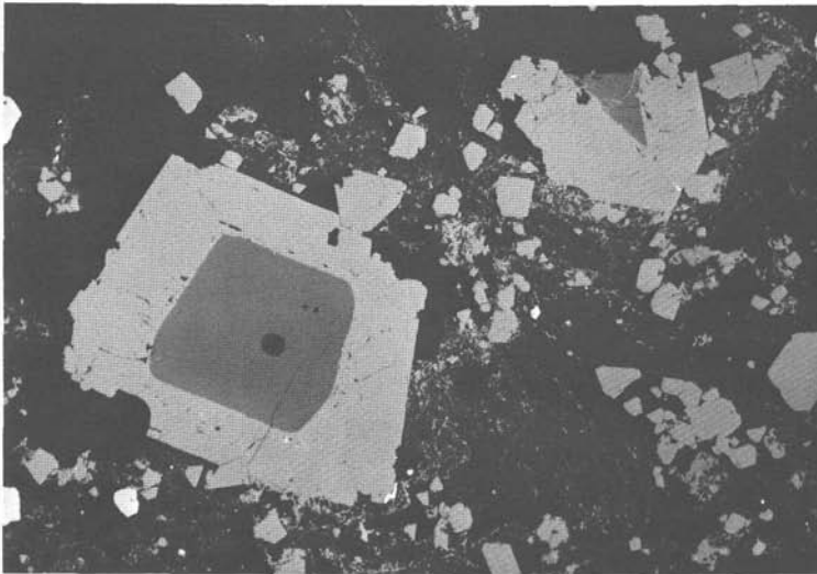
Abb. 28: Arzwaldgraben, Waldstein (Steiermark). Baryt-Gangart (fast schwarz), darin reichlich idiomorpher Magnetit (mittelgrau), der im Zentrum Chromit (dunkelgrau) als Einschluss, z. T. in vergleichbarer Kristallform, aufweisen kann. Neben kleinen Magnetit-Idiomorphen finden sich feinkörnige Rutil-Aggregate und -Züge (ebenfalls mittelgrau) sowie örtlich etwas Pyrit (lichtgrau) in der Baryt-Gangart. Anschliff, Vergr.: 150×
