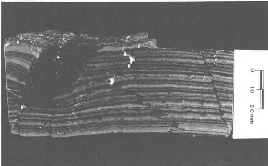
Abb. 8: Mežica, Graben-Revier, 11. Lauf, liegender Bereich des Riffes. Bleiglanz-Zinkblende-Dolomit-Rhythmit mit Load-casts an größerer, sammelkristallisierter Bleiglanz-Partie. (Probe freundlicherweise von Dipl.-Ing. Dr. Štruel zur Verfügung gestellt.)
