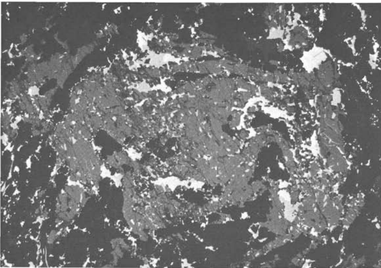
Abb. 15: Ramingstein (Salzburg). Synkinematisch gesproßter Granat (dunkelgrau) mit gedrehten, älteren Einschlußzügen („si“) von Quarz (schwarz) und Erzen (Bleiglantz – fast weiß; Zinkblende – lichtgrau; kleinste Tafeln von idioblastischem Ilmenit – ebenfalls lichtgrau). Randlich ist ein Übergang von einem Externgefüge („se“) „Erz-Gangart“ in ein Interngefüge „Erz und Gangart in Granat“ erkennbar. Entlang feinen, jüngeren Rissen kommt es im Granat zur Mobilisierung seiner alten Erz- und Gangart-Einschlüsse. Anschliff, Vergr.: 12×.
