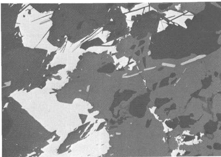
Abb. 11: Moosburg (Kärnten). Gruneritischer Amphibol (dunkelgrau) sprießt idioblastisch in älteren Bleiglanz (lichtgrau, fast weiß), läßt stellenweise außerdem asbestförmige Ausbildung erkennen (obere Bildhälfte) und ist mit porphyroblastischem Granat (licht dunkelgrau, rechte untere Bildhälfte) und Karbonat (dunkelgrau, verschiedene Töne) vergesellschaftet. Granat enthält Einschlüsse („si“) bzw. Verdrängungsreste von Quarz (dunkelgrau), Karbonat, Bleiglanz, idioblastischem Ilmenit (mittelgrau) und örtlich kleinste Graphit-Tafeln (mittelgrau bis schwarz). Anschliff, Vergr.: 150×.
