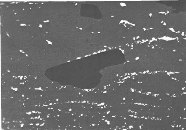
Abb. 34: Löffel-Graben, Vorau (Steiermark). Zinkblende (dunkelgrau), darin etwas Gangart (schwarz), weist Entmischung von Magnetkies (hellgrau) auf. Anschliff, Ölimmersion, Vergr.: 375X
