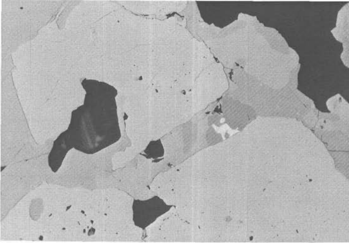
Abb. 14: Silberloch bei Ratten (Steiermark). Teilweise idioblastischer Pyrit (lichtgrau) mit Kupferkies (licht mittelgrau), Bleiglantz (Spur dunkler als Kupferkies), Magnetkies (mittelgrau), gediegen Gold (fast weiß) und Gangart (schwarz, z. T. durch Innenreflexe aufgehell). Risse im Pyrit werden von mobilisierten Sulfiden verheilt, der diese außerdem als Verdrängungsreste in seinen Idioblasten enthält. Anschliff, Ölimmersion, Vergr.: 245×.
