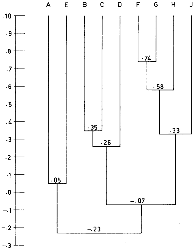
Abb. 8: Dendrogramm der Schwerminerale zur Clusteranalyse im R-mode (A Apatit, B Zirkon, C Turmalin, D Rutil, E Anatas, F Granat, G Hornblende, H Klinozoisit/Epidot, J Titanit).
