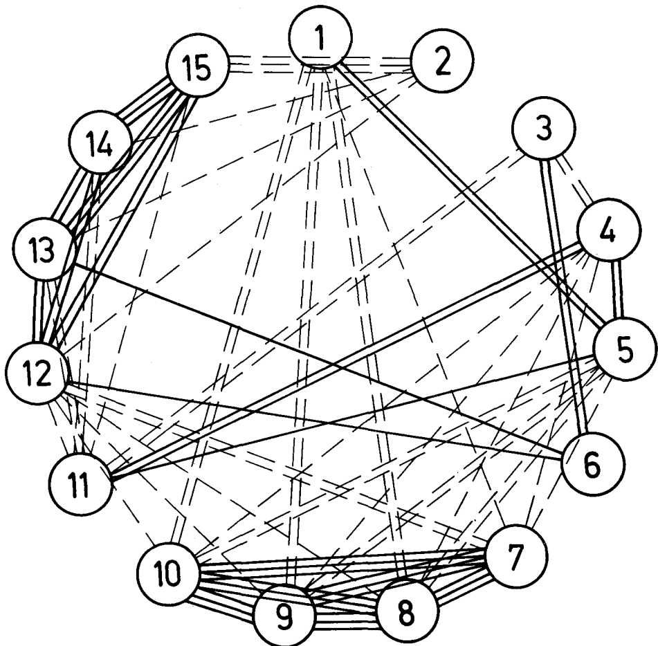
Abb. 3: Clusterdiagramm im R-mode der 15 aufgrund geochemischer Daten gebildeten Gruppen. Zuordnung 1—15 vgl. Tab. 2. (— r > .50 , - - r > .70 , ≡ r > .90 , die unterbrochenen Linien kennzeichnen die entsprechenden negativen Korrelationen)
