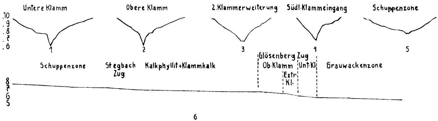
Fig. 4 Quer- und Längsprofile Liechtensteinklamm
