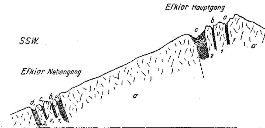
Fig. 6. Profil durch die Ausbisse des Efkiar-Haupt- und Nebenganges
