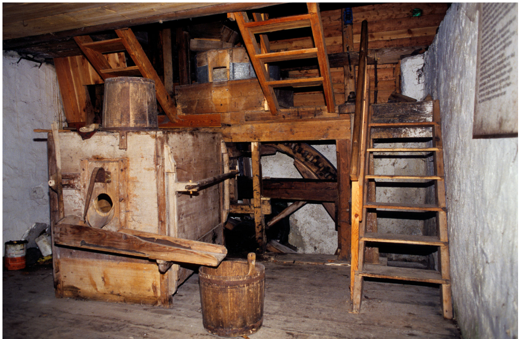
Blick in die Mahlstube der 1845 im Reifgraben bei St. Anton an der Jesnitz errichteten Weherberg-Mühle
