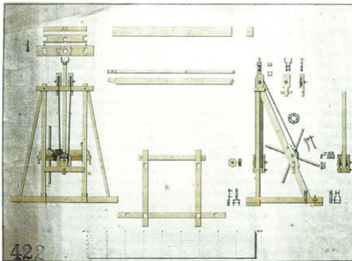
Plan eines Gerätes zum Umtopfen besonders großer und schwerer Pflanzen
