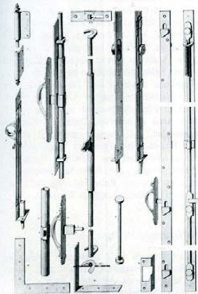
Beschläge für ein in Wien gebräuchliches nach innen aufgehendes Liggerfenster
