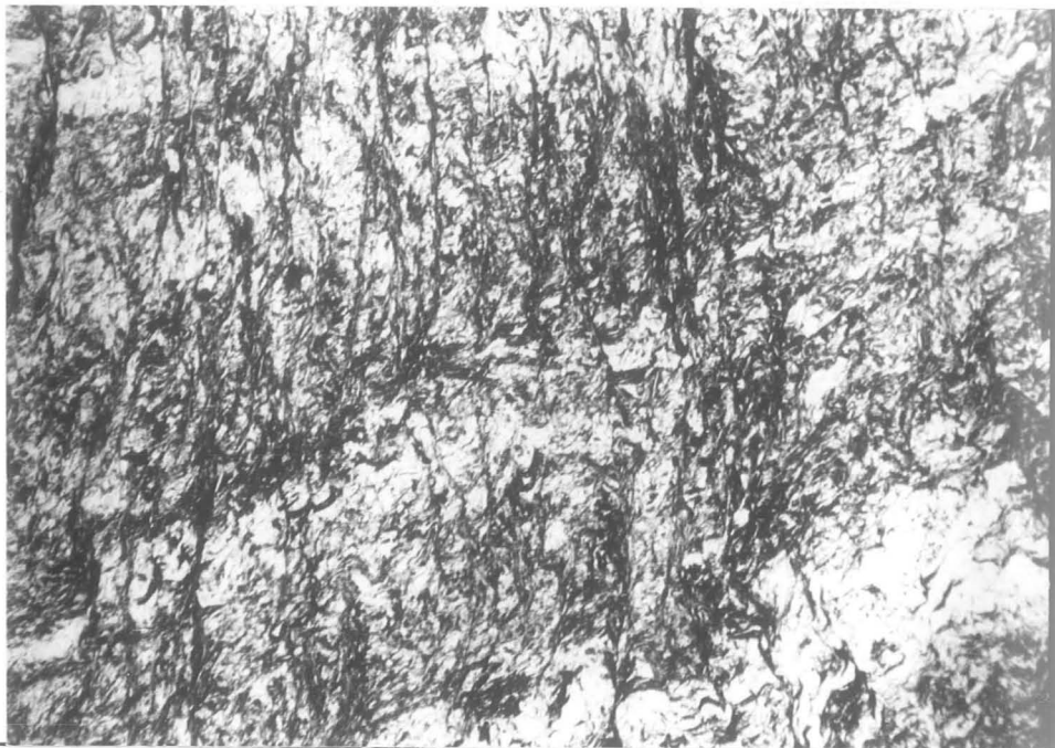
Abb. 1: P 10, Graphitphyllit, Vergr. ca. 12x, Nichols //. Graphitverteilung entlang dem sf_1 und einem älteren s.
