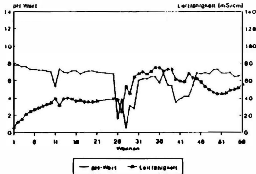
pH Wert und Leitfähigkeit der Perkolate
