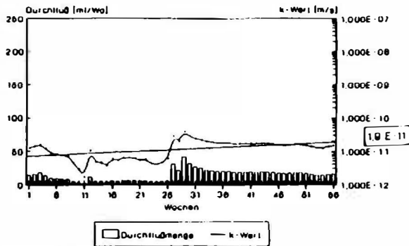
Durchfluß und k-Wert
