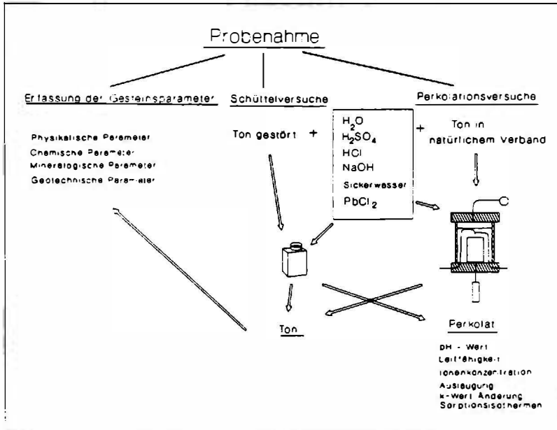
Abbildung 1: Ablaufschema der Untersuchungen
