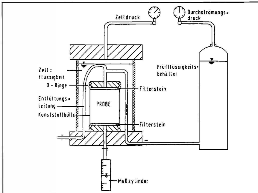
Abbildung 2: Schema einer Dreiaxial-Durchlässigkeitszelle
