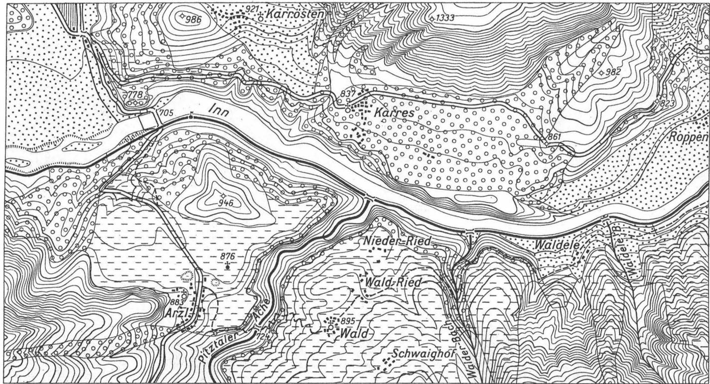
Fig. 2. Diluvialgeologische Kartenskizze des Inndurchbruchs von Karres 1 : 30.000.
