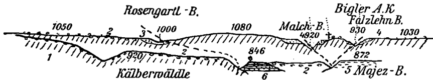
Fig. 5. Profil durch die Terrassenlandschaft westlich Imst.
