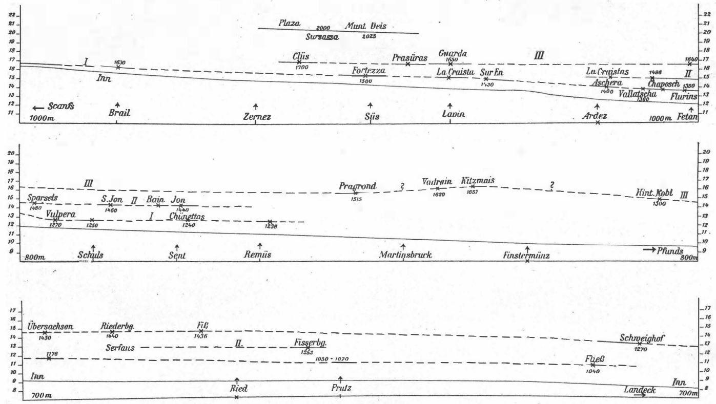
Fig. 1. Längsprofile der Inntalterrassen von Scans bis Landeck. Längenmaßstab 1 : 200.000, 4 1/2 mal überhöht.
