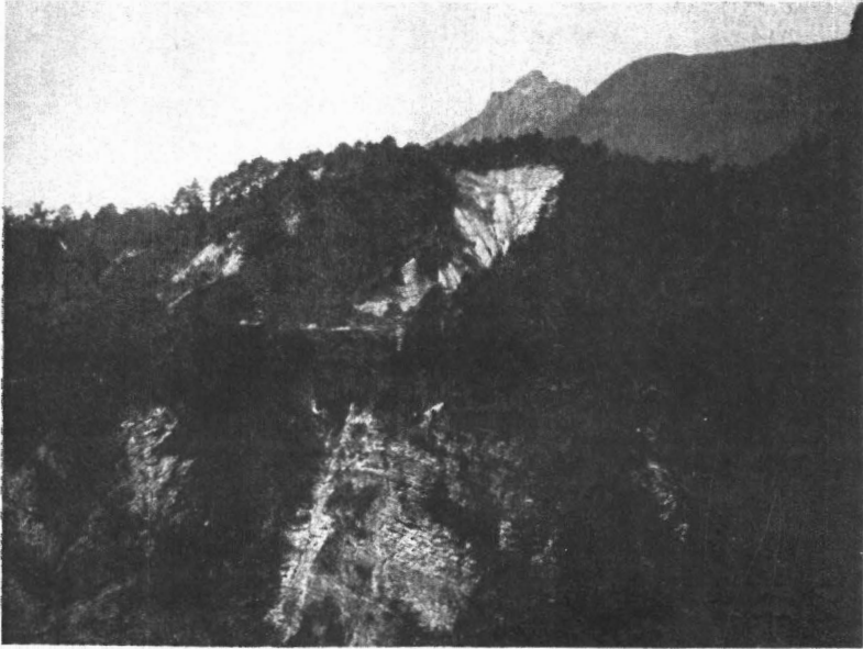
Abb. 1. Rechtes Gehänge der Salvesenschlucht. Schotter und Moräne über Hauptdolomit.
