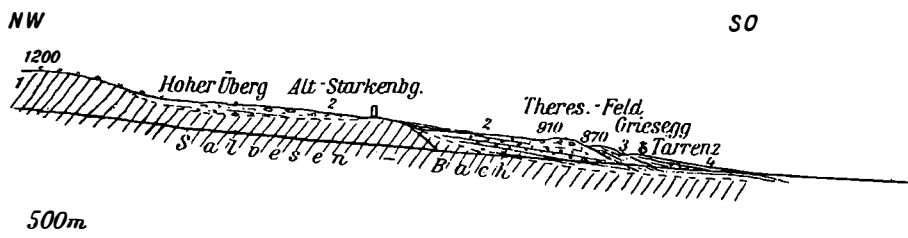
Fig. 7. Längsprofil durch die Salvesenschlucht
