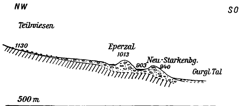
Fig. 6. Ufermoränen bei Starkenberg.
