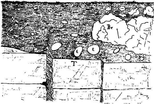
Fig. 2. Steinbruch bei Wemding (B). Die Tenuilobatus -Schichten (T) sind in der Richtung des Pfeiles geschrammt. K Keuperthon, D Geschiebe von braunem Jura, Br. brecciöser weisser Jura über der Schlißfläche.
