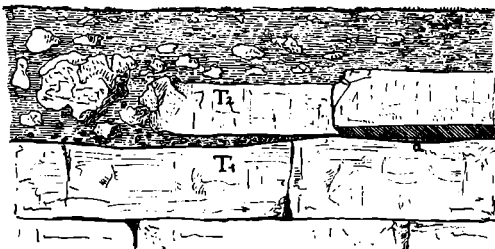
Fig. 3. Profil im Steinbruch von Wemding (A). T_1 Tenuilobatus -Bänke, auf der Oberseite geschrammt, T_2 überschobene Scholle desselben oder eines wenig höheren Niveaus, auf der Unterseite geschrammt.
