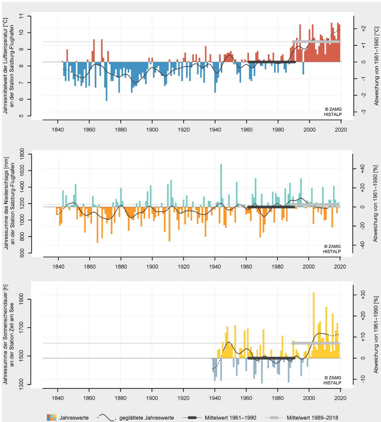
Abbildung 4: Zeitreihen der Jahreswerte für Lufttemperatur und Niederschlagssumme an der Station Salzburg-Flughafen sowie Sonnenscheindauer an der Station Zell am See ab Messbeginn bis 2019. Der Mittelwert im Referenzzeitraum 1961-1990 sowie der Mittelwert der letzten 30 Jahre sind jeweils mit dunkel- bzw. hellgrauen Balken gekennzeichnet.
