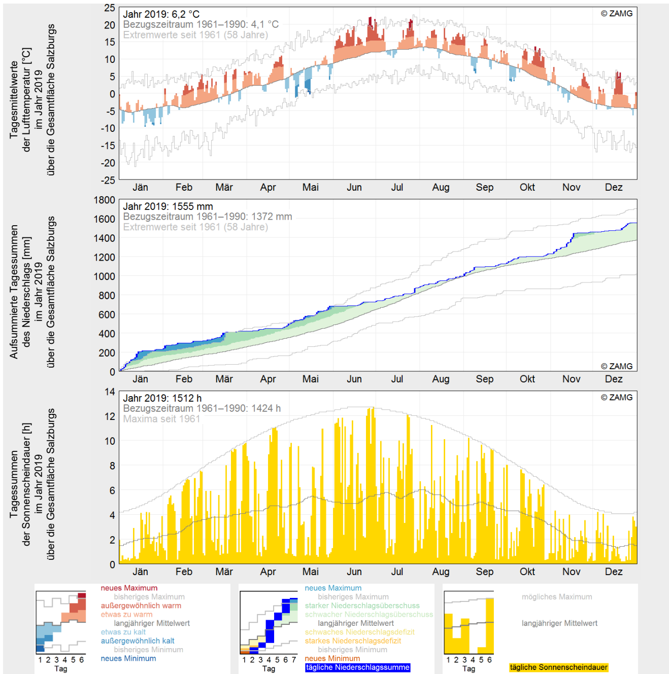
Abbildung 2: Jahresverlauf 2019 der Flächenmittel Salzburgs von Lufttemperatur, Niederschlagssumme und Sonnenscheindauer.
