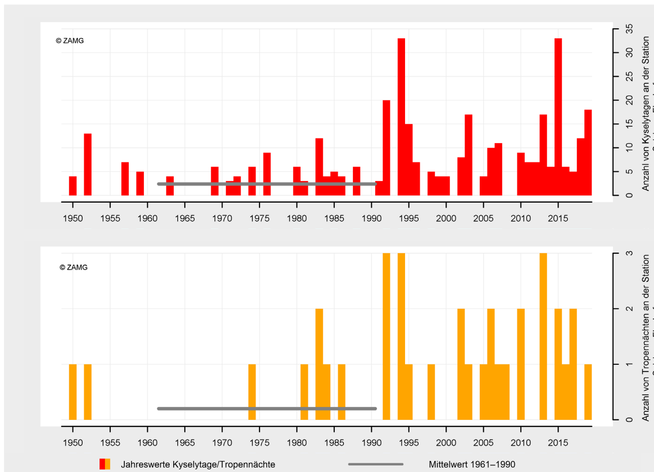
Abbildung 5: Zeitreihen der Anzahl von Kyselytagen bzw. Tropennächten an der Station Salzburg-Flughafen. Die grauen Balken stellen die jeweiligen Mittelwerte im Referenzzeitraum 1961-1990 dar.
