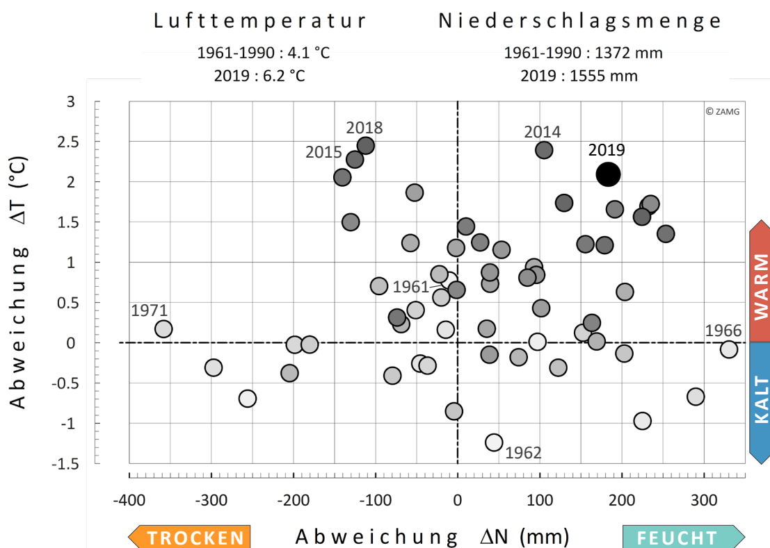
Abbildung 1: Gegenüberstellung der Jahressummen des Niederschlags und der Jahresmittelwerte der Lufttemperatur in Salzburg für die Jahre 1961 bis 2019. Die Jahreswerte sind als Abweichungen zum Referenzzeitraum 1961-1990 dargestellt und durch im zeitlichen Verlauf immer dunkler werdende Punkte gekennzeichnet.
