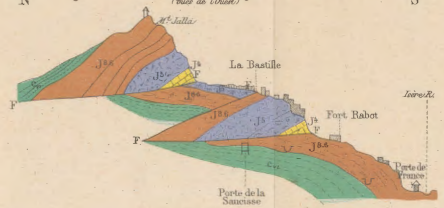
Fig. 3. Dislocations de la Montagne de la Bastille (rives de l'Ouest)
