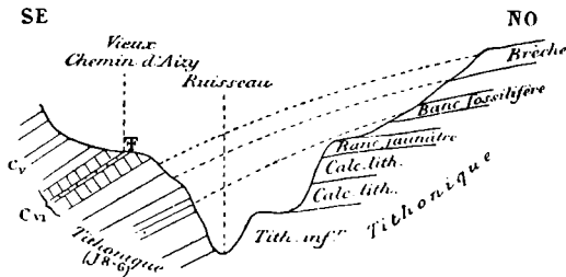
Fig. 2. — Coupe relevée près d'Aizy-sur-Noyarey.
