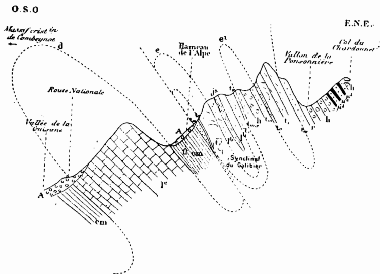
Fig. 9. — Coupe sur la rive dr. du vallon de l'Alpe.
