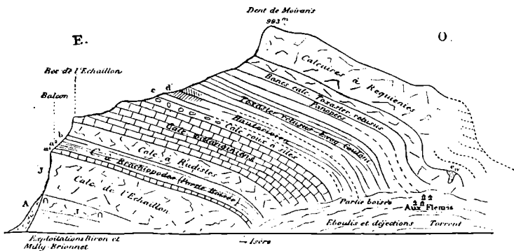
Fig. 3. — Coupe du promontoire de l'Échaillon (côté Nord) par W. Kilian et P. Lory.
