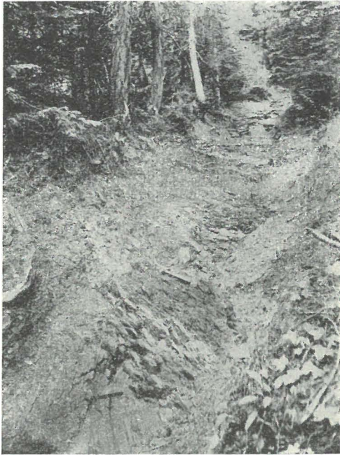
Fig. 3. Aufschluß in einem Hohlweg, der von der Fahrstraße Soboth—Krumbach, etwas östlich des Wirtshauses Lindner, gegen den Pirschlingkogel hinaufführt. Man sieht links unten die Schichtflächen einer obersten Schuppe (mit aufgemaltem Fallzeichen). Daneben scharf abschneidend die Schichtköpfe der nächsttieferen Schuppe. Im Hintergrunde, wo der Waldesschatten sich über den Weg legt, plötzlich wieder Plattenflächen, einer dritten Schuppe angehörig.
