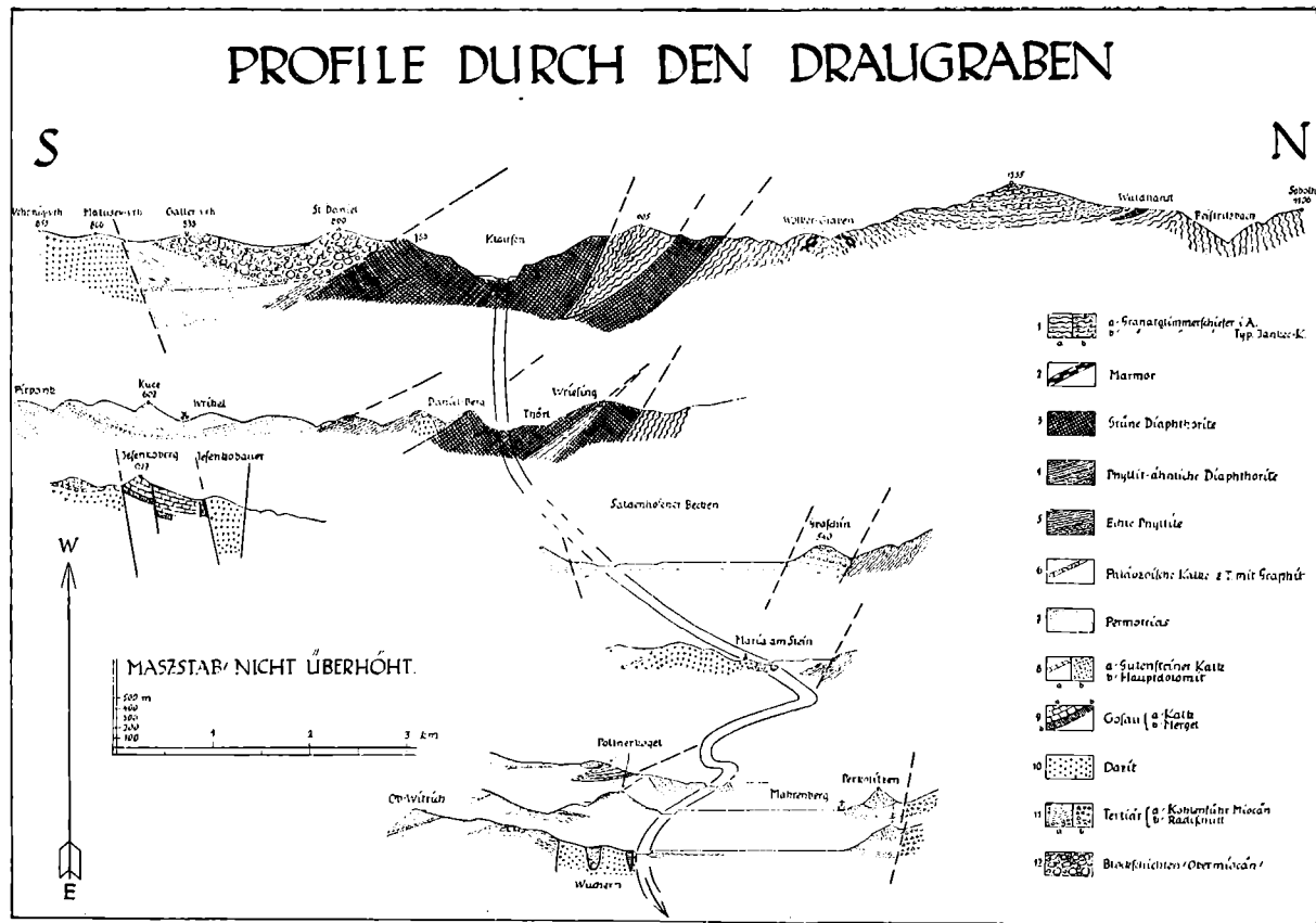
Fig. 5. Profile durch den Draugraben. Links Bachern, rechts Koralpe. Nicht überhöht. Man sieht (im obersten Profil), daß das Tertiär von St. Daniel keine Fortsetzung in der Koralpe hat.
