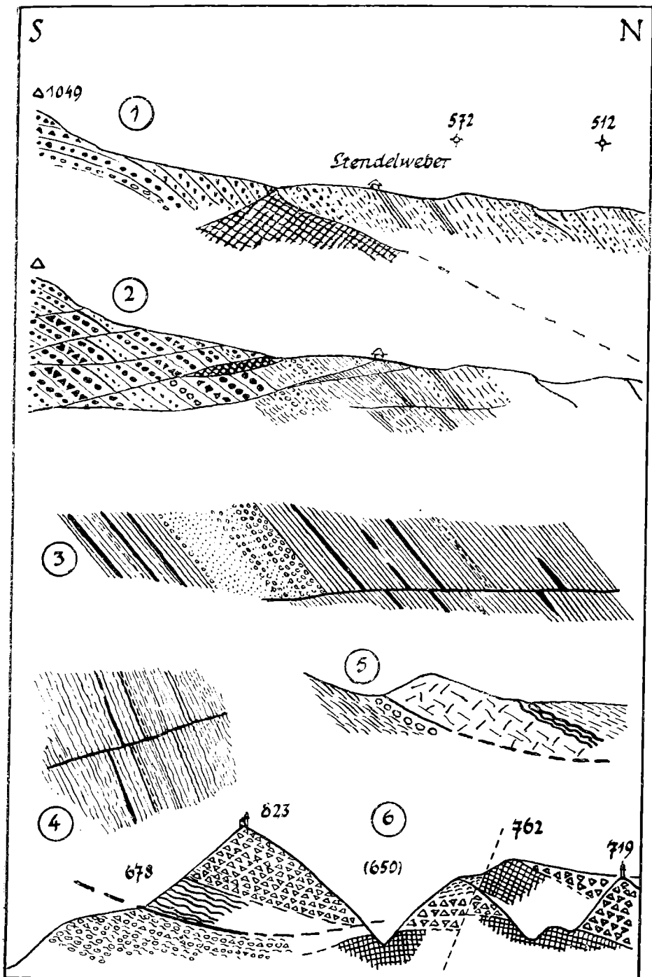
Fig. 4. 1. Profil Kapunerkogel (P. 1049) über Stendelweber, P. 572, P. 512 gegen Wasserleiter. Kopiert aus Winkler, Denkschriften, 101, Taf. I, Prof. 1. 2. Dasselbe Profil nach meiner Auffassung. 3. Überschiebung an der Straße Leutschach-Karnerberg. Umgezeichnet aus Winkler, Jahrb. G. R. A. 1913, p. 551, Fig. 2 (seitenverkehrt, damit gleiche Richtung mit den anderen Profilen). 4. Überschiebungen im Tertiär unter Hirzbauer. 5. Marmor-Glimmerschiefer-Linse, im Tertiär schwimmend. 600 m östlich von Bergweiß, in 590 m Seehöhe. 6. Profil Nauraschnik (P. 678), Hl. Drei König (P. 823), Oberer Radgraben (650), St. Anton (P. 719). — Kreuzrastr: Amphibolitdiaphthorit. Wellenlinien: Phyllit. Ringel mit kleinen Wellenlinien: leicht metamorphes Radkonglomerat. Dreiecke: frischer Radenschutt (einige feinsandige Lagen nicht ausgeschieden).
