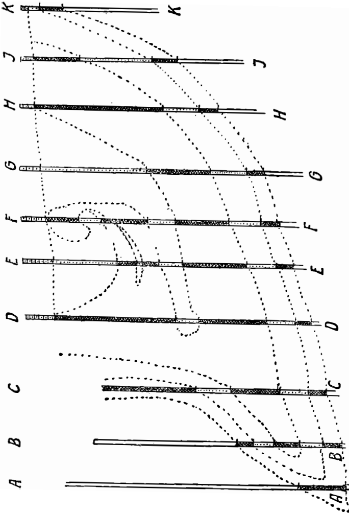
Fig. 3. Schematische Einschaltung von Bohrprofilen in die Scholle IV. Die einzelnen Profile entsprechen den Buchstaben der Fig. 1.
