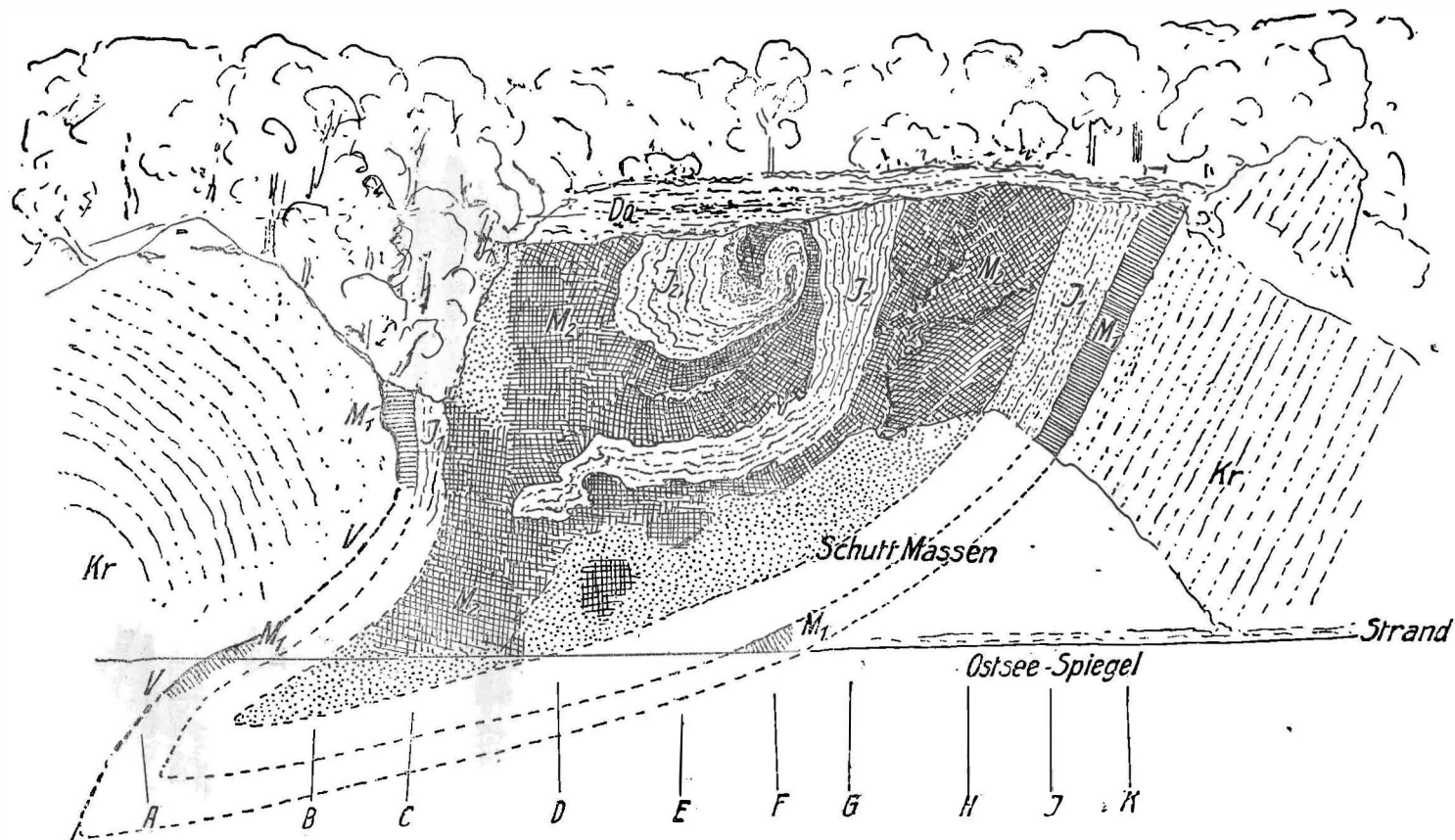
Fig. 1. Profil der Diluvialscholle IV am Lenzer Bach bei Saßnitz, rechts der liegende, links der hangende Flügel der Mulde. Kr oberes Miokäen, durch Flintebänke geschichtet. M 1 unterster Geschiebemergel, J 1 unterstes Interglazial, M 2 zweiter Geschiebemergel, J 2 zweites Interglazial. Do diskordant darüber liegende Schichten des jüngeren posttektonischen Diluviums, wahrscheinlich zu deren jüngsten Relikten gehörig. V Verwerfung. Die z. T. bewachsenen oder durch Gehängeschutt bedeckten Teile von M 2 punktiert. Verkleinerung etwa 1/500. Die Buchstaben A—K beziehen sich auf die Profile der Figur 3.
