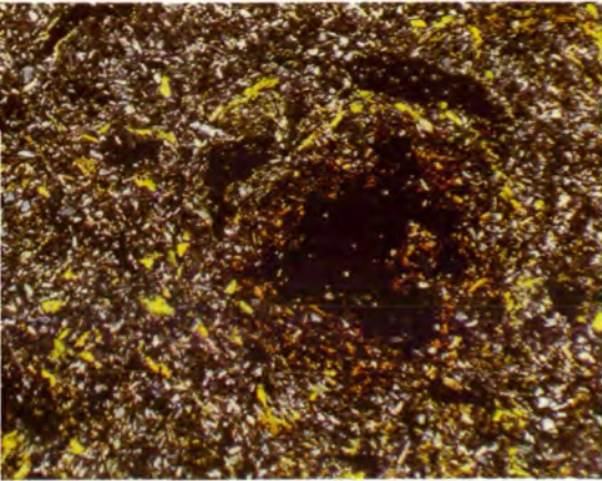
Abb. 5: B 1 -Horizont bei 40 cm Dichtes, noch hohlraumreiches, feinkörniges Mineralgefüge, bestehend aus Quarz, Feldspat und Glimmerschüppchen, mit viel Bindesubstanz, die teils gut ausgeflockt und teils schlierig zusammengeballt ist. Dabei zeigen junge Toneisenhydroxide hellgelbe Farbe und starke Doppelbrechung, während alternde Gele dunkelrotbraun und nicht doppelbrechend aufscheinen.
