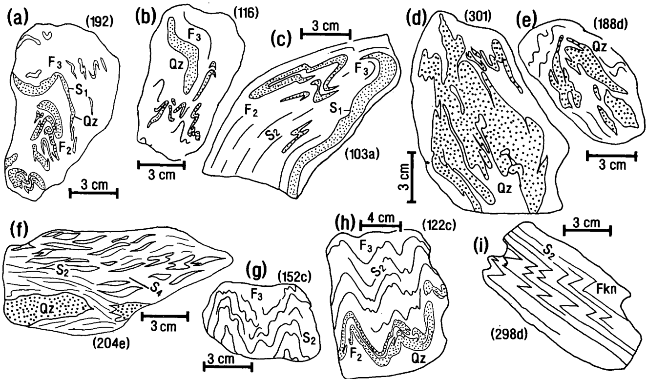
Abb. 8. Faltenstrukturen in Phylliten aus dem Thurntaler Komplex. Quarzlagen sind gepunktet dargestellt. a-e, g und h zeigen Schnitte senkrecht zur Knickfaltenachse F_3 ; i zeigt einen Schnitt senkrecht zur Knickfaltenachse. Alle Strukturen sind lagerichtig (links ist NNW, rechts SSE) gezeichnet. f zeigt einen Schnitt parallel zur Lineation (links ist WSW). Bei allen Handstücken handelt es sich um Phyllite.
