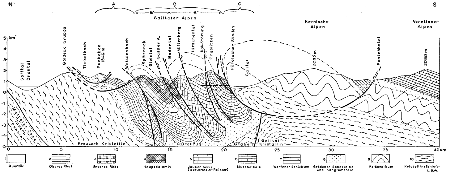
Abb. 4: Übersichtsprüfil der zentralen Gailtaler Alpen
