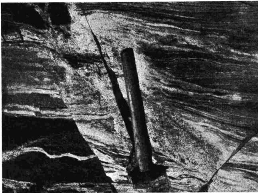
Abb. 15: Saurer Tonalitgranit im Quer- und Parallelkontakt mit altkristallinen Schiefergneisen. Ein Beispiel in Miniatur für immigrative Platznahme magmatischer Massen und die Entstehung von Parallelkontakten. Maltatal, Hochalmspitzgebiet.
