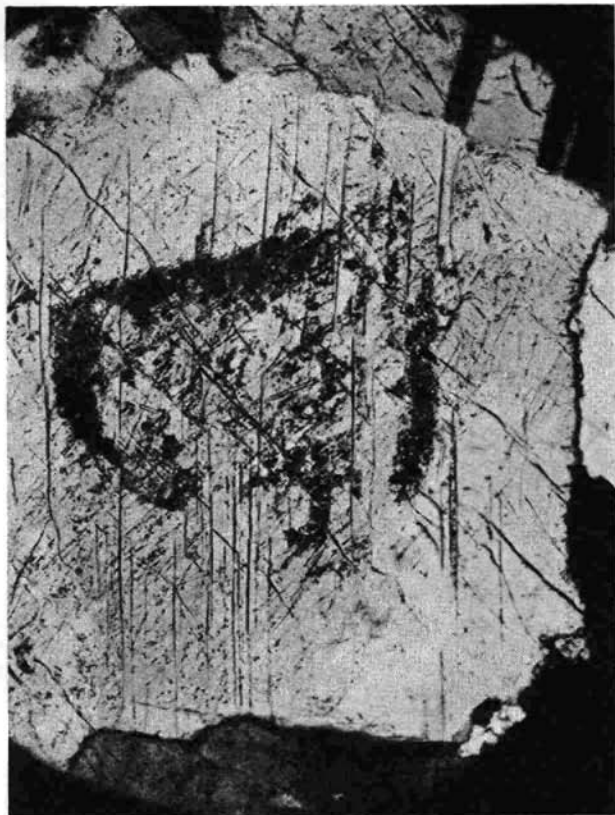
Abb. 35: Gerüstplagioklas mit feinkörniger Mikrolithenfüllung im Bytownitbereich. Kerngerüst (bzw. Kernring) wird durch beginnende Mikrolithenbildung nachgezeichnet und erzeugt gleiche Gefügebilder in Anfängen, wie sie in den Plagioklasen der Tauern-Tonalite vollendet sind (vgl. Abb. 16). // Nicols, etwa 80fache Vergrößerung.
