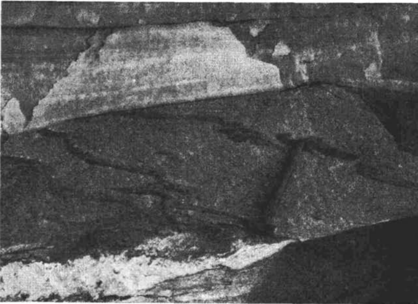
Abb. 11: Metatexit bis Anatexit mit jüngeren Apliten; das Ende des Hammerstieles zeigt auf ehemalige Biotitplagioklasgneis-Lage, die sich in stark erweichtem Zustande in einzelne Schlieren auflöst. Das Bild soll eine von mehreren Möglichkeiten zeigen, auf welche Weise „basische Putzen“ entstehen. Gletschervorfeld Hornkees, Oberer Zemmgrund (Zillertal).
