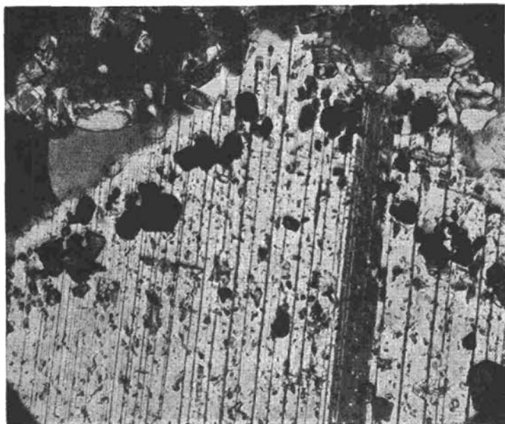
Abb. 30: Gefüllter Albit a mit Granatmikrolithenzone an der Grenze gegen ungefüllten Albit n . Schräge Nicols, etwa 200fache Vergrößerung.
