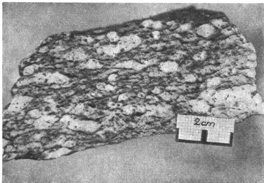
Abb. 7: Augengranitgneis. Mittleres Obersulzbachtal, orogr. links, Krauskar, Groß- venediger.
