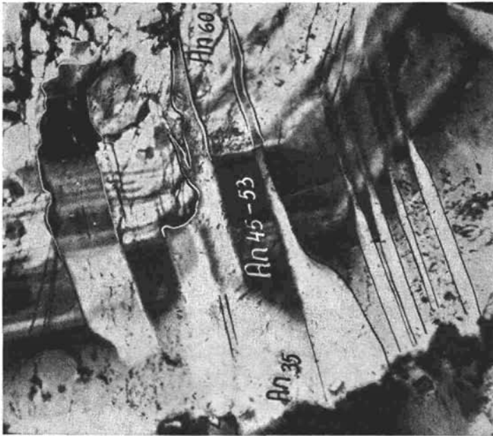
Abb. 38: Ausschnitt aus einem Tonalitplagioklas mit Kerngerüst ( An_{60} ) und Hüllplagioklas ( An_{35-53} ). Albitzwillingslamellen (Konturen nachgezeichnet) verändern sich bei Eintritt in basischere Zonen und verlieren sich schließlich ganz im Gerüstkern. Gekreuzte Nicols, etwa 100fache Vergrößerung.
