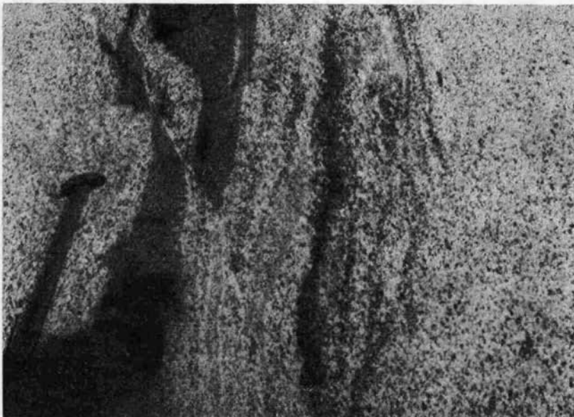
Abb. 6: Metatexit bis Anatexit durch Tonalitimmigration parallel s der Biotit-plagioklasgneise und weitgehende Auflösung des alten Gefügeverbandes. Abb. 4 kann als Anfangsstadium dieser Entwicklung verstanden werden. Obersulzbachtal, Gletscherschliffe vor der Gletscherzunge des Obersulzbachkeeses, Großvenediger.
