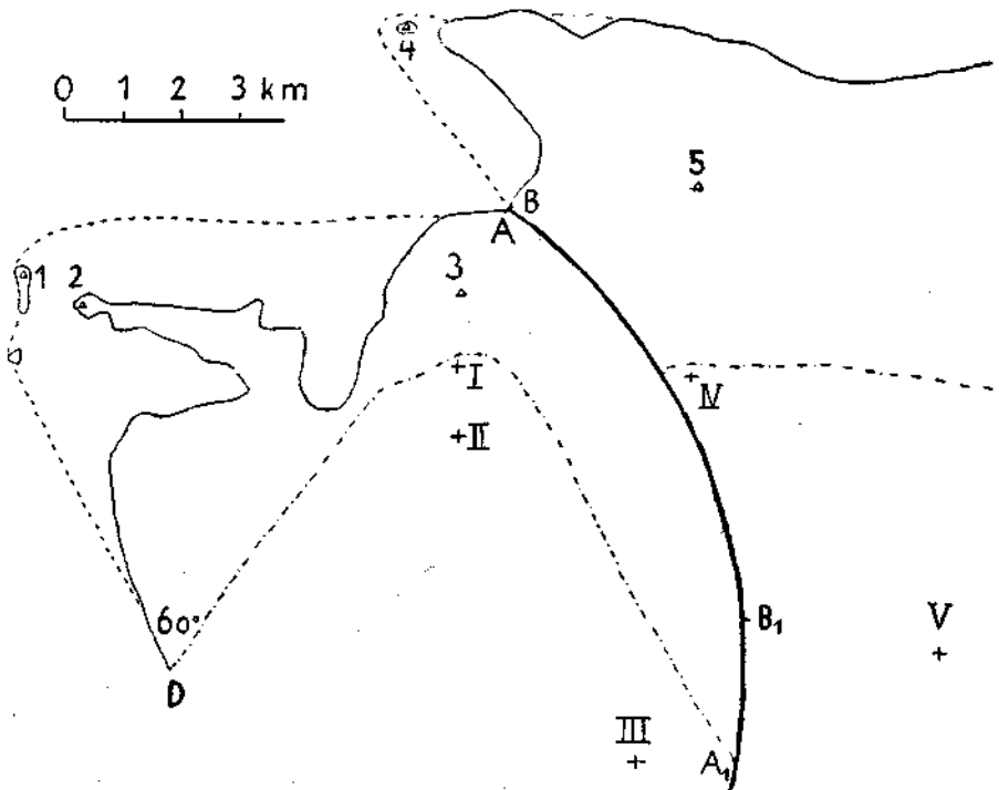
Abb. 2. Bewegungsschemata der Achantaler und der Guffert-Schubmasse.
