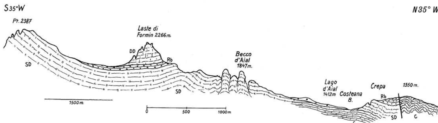
Fig. 49. Laste di Formin—Crepa di Belvedere (i. M. 1 : 30.000).
