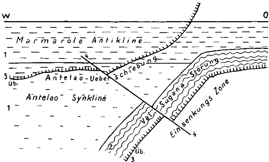
Fig. 42. Kartenschema eines Beispiels der tektonischen Vorgänge im Val Cadore. 1. Bildung der Haupt-Schollen mit O-W Faltenbau. 2. Aufwölbung der Val Sugana Störungszone. 3. Entwicklung einer S und SO Überschiebung (Üb) am Südrand der Marmarole-Scholle und Vordringen derselben ins Gebiet der Antelao Synklinė; Überschiebung in der Val Sugana Störungszone von W nach O gerichtet. Zugleich senkrechte Quersprünge und Klüftungen in den Schubmassen. 4. Mehrfache weitere Entwicklung von lokalen Falten, Senkungen und Quer- und Diagonalbrüchen. Wichtigste davon im Cadore-Tal der NW-SO Bruch im unteren Val d'Oten (in dem Schema eingetragen), der sowohl die Antelao wie die Val Sugana Störungszone nach SO verschiebt.
