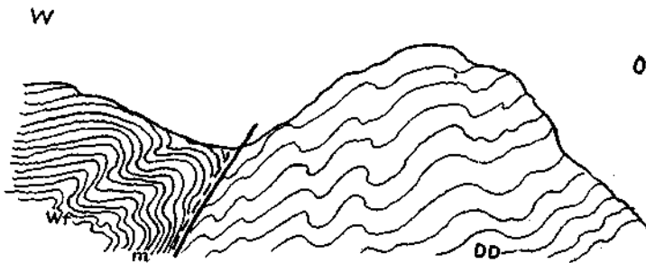
Fig. 40b. Hauptstörung im Piave-Tal bei Cantoniera, 839 m. Zwischen Werfener Schichten ( Wf ) an der Störung mylonitisiert ( m ) und Dachsteindolomit ( DD ). Die Werfener Schichten sind steil auf den gesenkten Dachsteindolomit geschoben.
