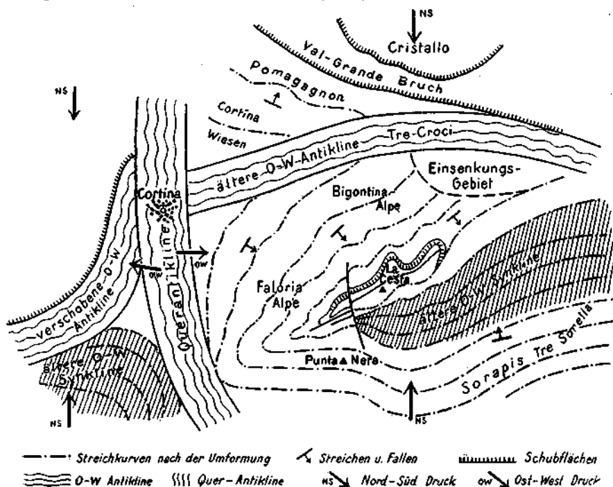
Fig. 21. Karte der Umformung des O W Streichens infolge von Querfaltung, schematisch dargestellt für das La Cesta-Gebiet.
