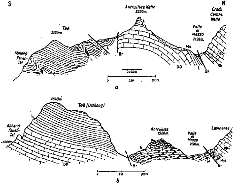
Fig. 48. Zwei parallele Querprofile durch die Antruilles Kette.
