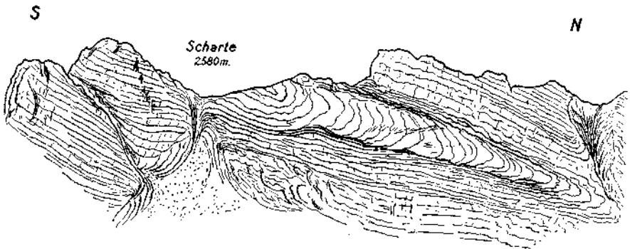
Fig. 14. Ansicht der liegenden Falte im Liaskalk des Felssporns von Col Freddo; von SO gesehen.
