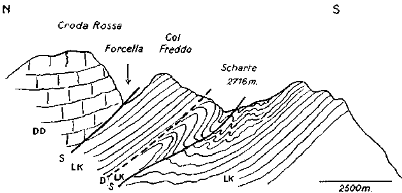
Fig. 13. Die Schubflächen ( S ) von Croda Rossa und Col Freddo (i. M.: 1:12.500). LK = Liaskalk. DD = Dachsteindolomit. D = Faltendiskordanz.
