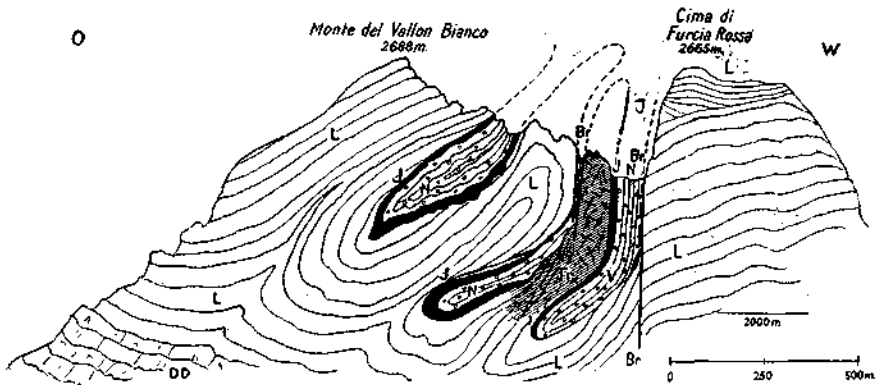
Fig. 45. Profil von Monte del Vallon Bianco.
