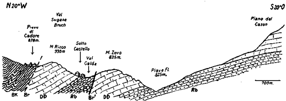
Fig. 36. Lage von Pieve di Cadore unmittelbar an der Val Sugana-Störungszone. Br = „Val Sugana-Linie“ zwischen dem Oberperm-Bellerophonkalk ( BK ) im W und dem gesenkten Dachsteindolomit ( DD ) im Osten. Br' = Nebenstörung zwischen Raibler Schichten ( Rb ) und Dachsteindolomit (i. M. 1 : 33.000).
