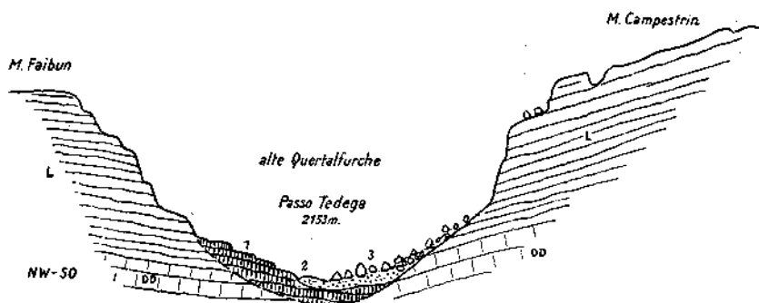
Fig. 44. Passo Tedega — eine alte Quertalfurche.
