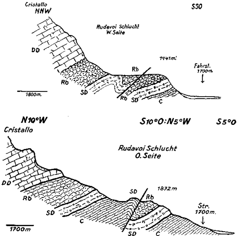
Fig. 11—12. Fortsetzung der M. Cristallo-Störungszone nach O im Rudavoi-Gebiet. DD = Dachsteindolomit. Rb = Raibler Schichten. SD = Schlerndolomit. C = Cassianer Schichten. Str = Fahrstraße.
