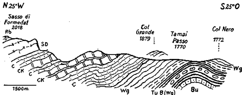
Fig. 53. Querschnitt Passo Tamai—Sasso di Formedal.
