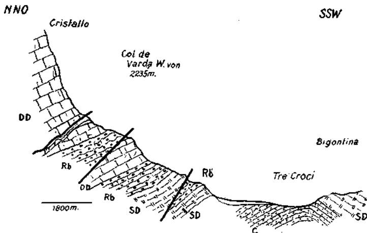
Fig. 10. Profil durch die Störungszone am Südhang des M. Cristallo. Kleine Keile Raibler Schichten im Dachsteindolomit (DD) der Steilwand. Überschiebungen: die obere schneidet durch Col de Varda—Raibler Sch. (Rb) auf Dachsteindolomit (DD); untere (Val Grande Bruch), Schlerndolomit (SD) auf Raibler Sch.
