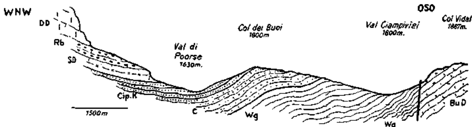
Fig. 24. Profil des Col dei Buoi. Im W Cresta Giastellin, im Osten Col Vidal. Einbruch der Schichtfolge Dachsteindolomit (DD)—Wengener Schichten (Wg), gegen den Buchensteiner Dolomit (BuD) von Col Vidal östlich des Bruchs. Rb = Raibler Schichten. SD = Schlerndolomit. Cip = obere Cassianer Gipfalkalke und Tuffe. C = Cassianer Schichten (i. M. 1 : 25.000).
