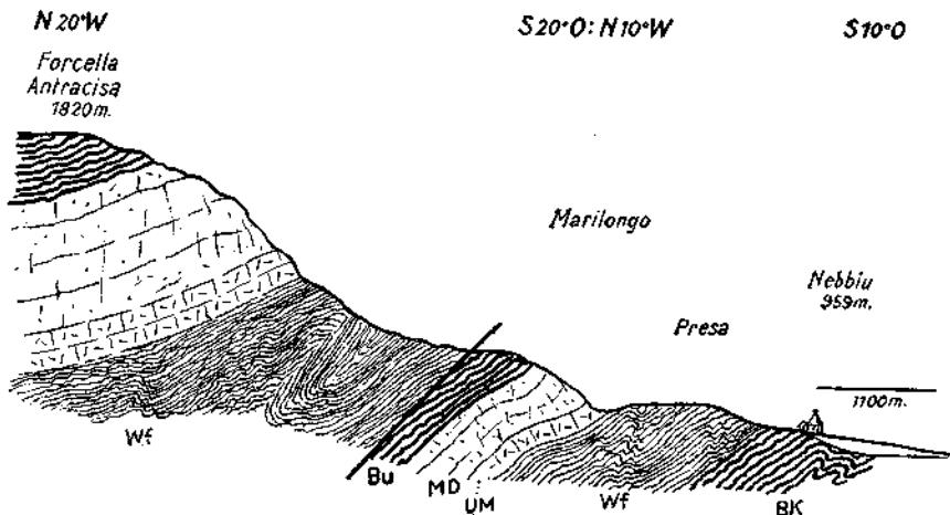
Fig. 29. Gefaltete Werfener Schichten gegen Buchensteiner Schichten aufgeschoben. BK = Bellerophonkalk. Wiederholung der Schichtfolge Werfener Schichten (Wf); Unterer Muschelkalk (UM); Mendoladolomit (MD); Buchensteiner Schichten (Bu); (i. M. 1 : 25.000).
