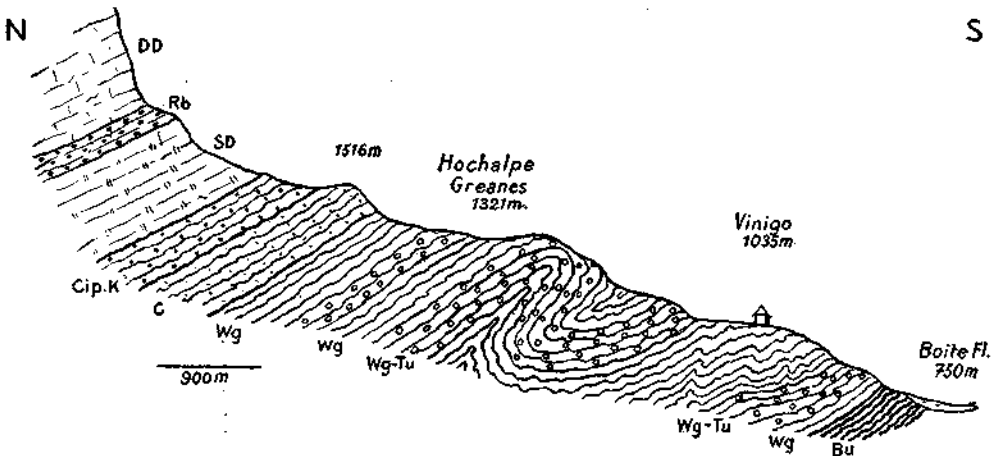
Fig. 32. Gefaltete Wengener Tuffe im Südhang des M. Antelao oberhalb Vinigo. DD = Dachsteindolomit. Rb = Raibler Schichten. SD = Schlerndolomit. CK = Oberer Cassianer Cipitkalk und Tuff. C = Cassianer Schichten. Wg = Wengener Tuffmergel- und Sandsteine. WgTu = Wengener Tuffe und Tuffkonglomerate. Bu = Buchensteiner Pietra verde und Plattenkalke (i. M. 1 : 25.000).
