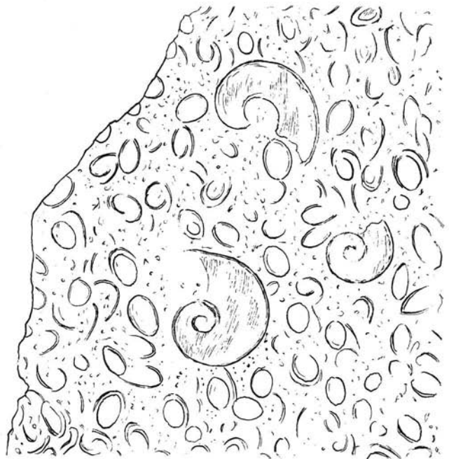
Fig. 6 (10×). „Ostracodenkalk“ mit Ostracoden erfüllt und mit einigen Bellerophon Jugendformen.
