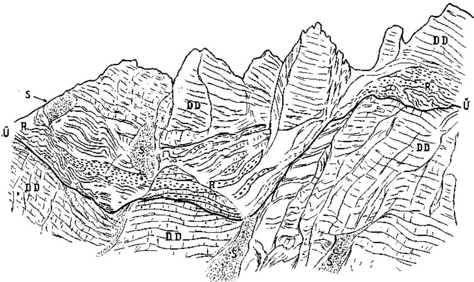
Fig. 9. Skizze der oberen Überschiebung (Ü) am Südhang des M. Cristallo. Gestörte Raibler Schichten (R) auf Dachsteindolomit (DD) überschoben. Rechts eine Queraufbiegung der Überschiebung. S = Schuttrinnen.
