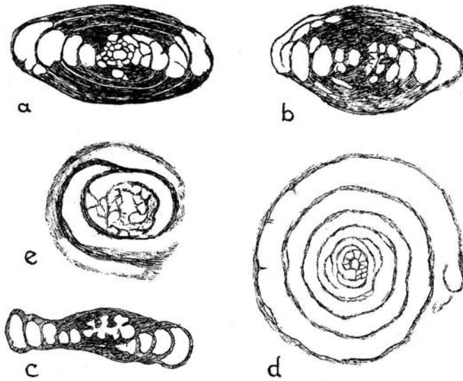
Fig. 5 (40×). Fusulinella Itoi , Osawa. Längs- und Querschnitte a—e
