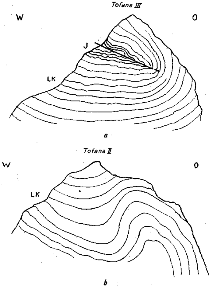
Fig. 46. Gipfelfaltungen in Tofana II und Tofana III.
