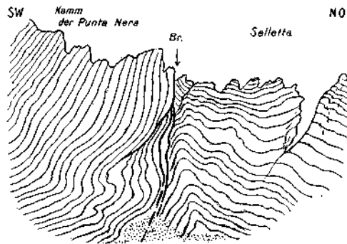
Fig. 20 a. Der „Selletta-Bruch“.
