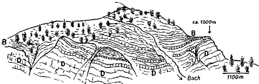
Fig. 8. Ansichtsskizze des Übergangs von Buchensteiner Kalk, Mergel und Tuff (B) in Dolomittfazies (D). Bacheinschnitt NW San Marco di Palus, Val Ansiei.
