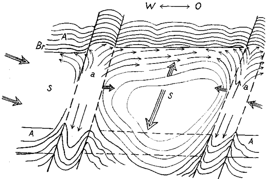
Fig. 41. Kartenschema der Umformung von älteren O-W Falten durch das Eingreifen jüngerer Querfallen.
