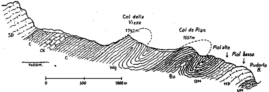
Fig. 52. Profil durch den Südhang des Zoppe Gebietes.
