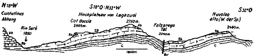
Fig. 43. Profil Lagazuoi—Nuvolao.
