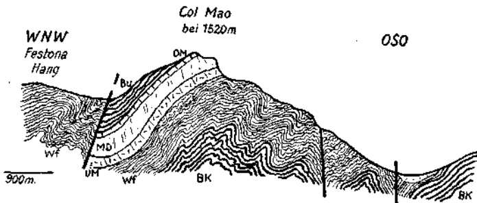
Fig. 30. Zerschnittene Falte im Westhang von Col Mao westlich von Nebbiu. Die Werfener Schichten ( Wf ) des Festona Hanges sind gegen die jüngere Schichtfolge am Westhang von Col Mao aufgeschoben.
