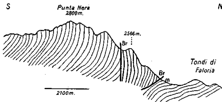
Fig. 20 b. Querschnitt Faloria—Punta Nera (i. M. 1 : 25.000). Am Westende der La Cesta-Kette westlich des Selletta-Querbruches. Br = Brüche. M = Mylonitzone der Terrasse.
