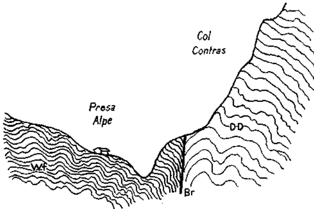
Fig. 40a. Querbruch im nördlichen Teil des Col Contras. DD = Dachsteindolomit. Wf = Werfener Schichten. Br = Bruch. Der Bruch streicht NNW—SSO.
