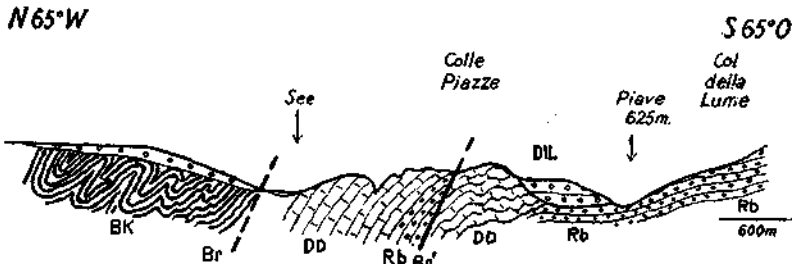
Fig. 37. Die Val Sugana-Störungszone im Piave-Tal unterhalb Calalzo. Br = Val Sugana-Linie. Br' = Nebenstörung. DD = Dachsteindolomit. Rb = Raibler Schichten. BK = Bellerophonkalk. DIL = Diluvialbreccien (i. M. 1 : 12.500).
