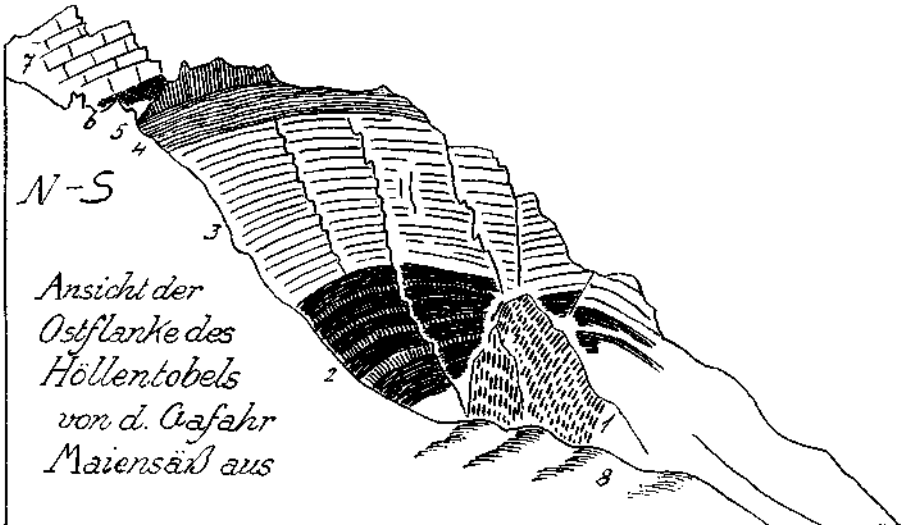
Fig. 7. 1 = Buntsandstein, gut erhalten. 2 = Partnachsichten. 3 = Arlbergsschichten. — Raibler Schichten: 4 = Lunzer Sandsteine. 5 = Kalk, Dolomit. 6 = Gipsrauwacken. — 7 = Hauptdolomit. 8 = Moränenwälle.
