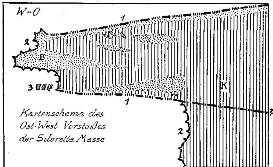
Fig. 14. 1 = steilstehende Verschiebungsfläche. 2 = flachliegende Schubfläche. 3 = Schubschollen. K = Silvrettakristallin. B = Auflagerungen von Verrucano-Buntsandstein und jüngeren Schichten. Zu Fig. 14 stellt Fig. 15 einen schematischen Längsschnitt dar.
