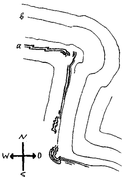
Fig. 4. Gelenk in den Fleckenmergeln der Südsperrre des Spullerseees. a = weite Kalzitklüfte. b = Schichtfugen der Liasfleckenmergel.
