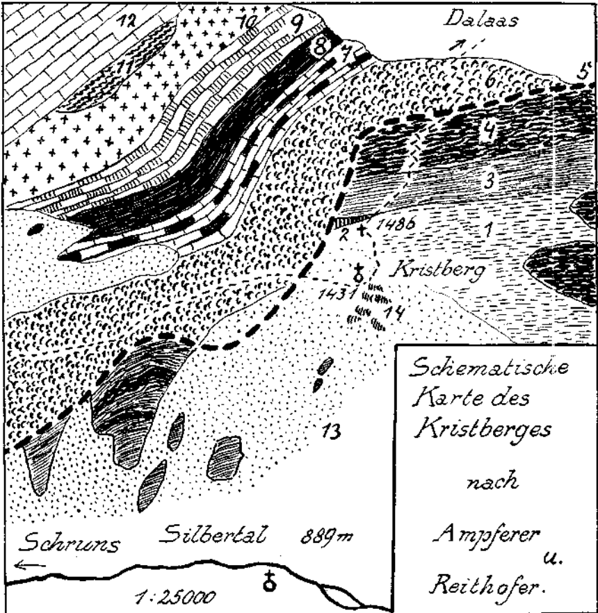
Fig. 8. 1 = Schiefergneis. 2 = Quarzit. 3 = Phyllitgneis und Glimmerschiefer. 4 = Muskovitgrauit-gneis. 5 = Grenze des Kristallins mit Karbonresten. 6 = Buntsandstein und Verrucano. 7 = Muschelkalk. 8 = Farnachsen-schichten. 9 = Arlberg-schichten. 10 = Raibler Schichten. 11 = Gips-lager. 12 = Hauptdolomit. 13 = Moränen. 14 = Alte Bergwerkshalden.
