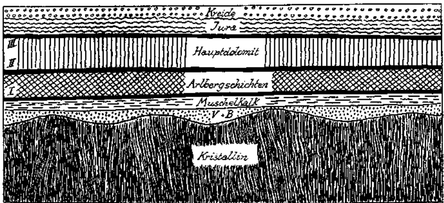
Fig. 17. Schema der Ausgangsstellung der Silvrettamasse und ihrer Sedimentdecke für die großen S-N-Bewegungen. Hauptgleichhorizonte: I = Partnachschichten, II = Raibler Schichten, III = Kössener Schichten.
