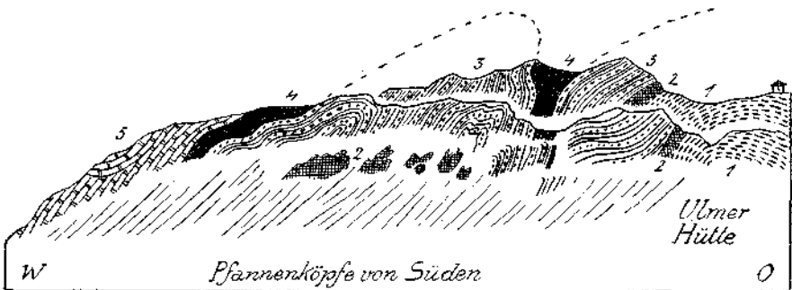
Fig. 3. 1 = geschieferter Verrucano. 2 = Rauhwacke. 3 = Muschelkalk. 4 = Partnachschichten. 5 = Arlbergsschichten.
