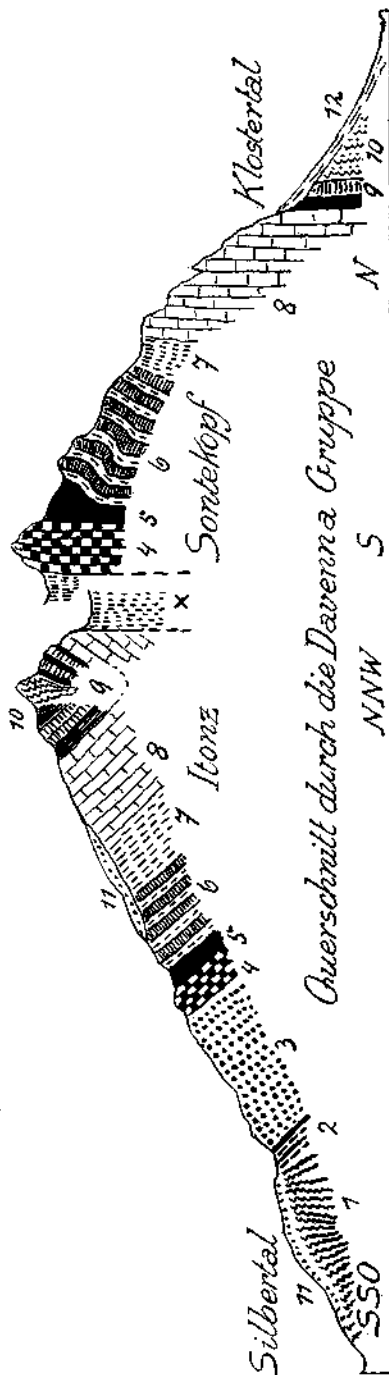
Fig. 9. 1 = Phyllitgneis und Glimmerschiefer, 2 = Karbonzone, 3 = Verrucano und Buntsandstein, 4 = Muschelkalk, 5 = Parlanaschichten, 6 = Aribergschichten, 7 = Raibler Schichten, 8 = Hauptdolomit, 9 = Kössener Schichten mit Oberrätikalk, 10 = Lösshornsteinkalke am Honz, 11 = Liasstockmergel im Klostertal, 12 = Moränen, 13 = Schattbalden, X = große Masse von stark ausgewalztem Gips der Raibler Schichten.
