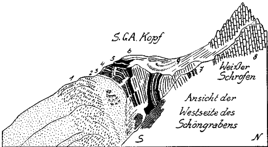
Fig. 1. 1 = Verrukano. 2 = Buntsandstein. 3 = Raubwacke. 4 = Muschelkalk. 5 = Partnachschichten. 6 = Arlbergschichten. 7 = Raibler Schichten. 8 = Hauptdolomit. 9 = Moränenwälle. 10 = Rutschungen.
