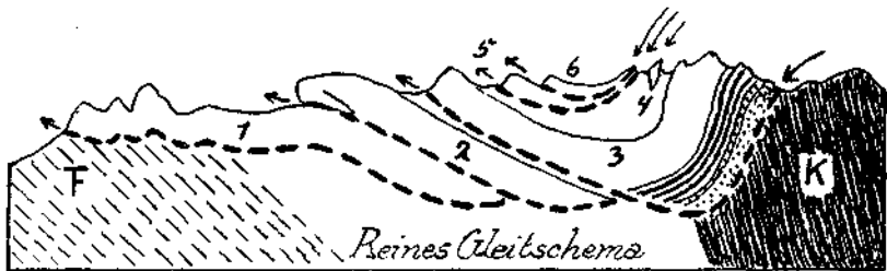
Fig. 19. 1-2-3-4-5-6 = lauter Gleitdecken. K = Altcrystallin. F = Flysch.
