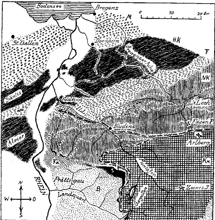
Fig. 25. Kr = Silvrettakristallin. NK = nördliche Kalkalpen. S = Salzfuhdecks. Fa = Falkraidecks. B = Bündner Schiefer. F = Flysch. HK = Schweizer Kreide. M = Molasse. ← = junge O-W-Verschubslinie. Schematische tektonische Karte von Vorarlberg.
