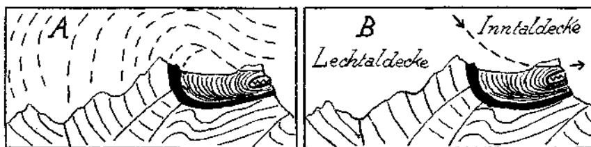
Fig. 22. A = Erklärung durch Überfaltung und Ausquetschung von Kössener Schichten + Oberrätikal-Plattenkalk. B = Erklärung durch Reliefüberschiebung der Inntaldecke.
