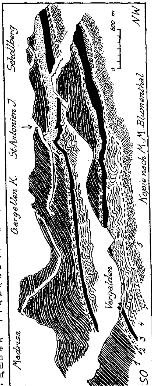
Fig. 16. 1 = Silvrettkristallin, 2 = Arosazone, 3 = Sulzfluhdecke, 4 = Falknisdecke, 5 = Bündner Schiefer. Sammelprofil für das Gargellenfenster. Kopie nach M. M. Blumenthal
